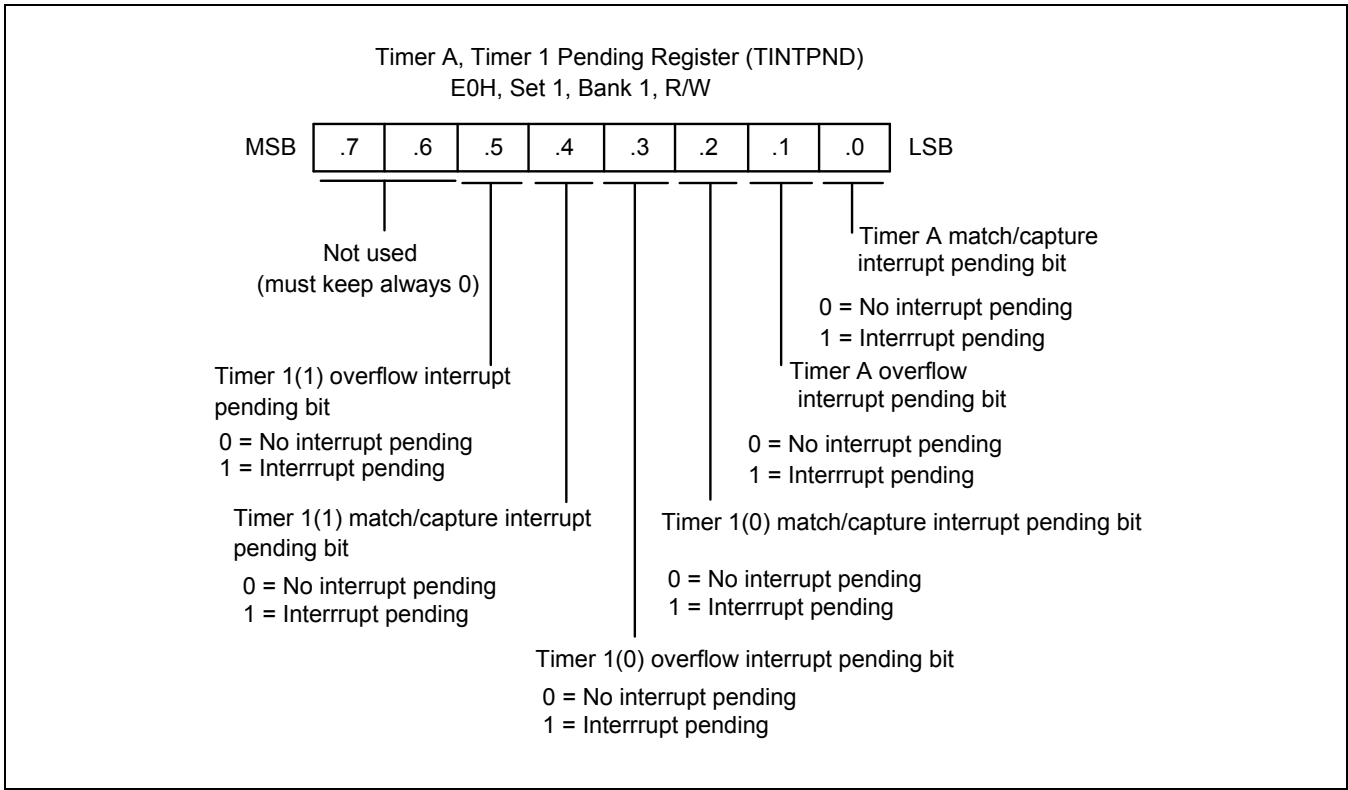
图 12-2 Timer A, Timer 1(0, 1) 中断标志寄存器 (TINTPND)
