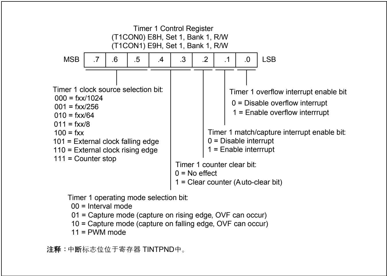
图 12-1 Timer 1(0,1) 控制寄存器 (T1CON0, T1CON1)
