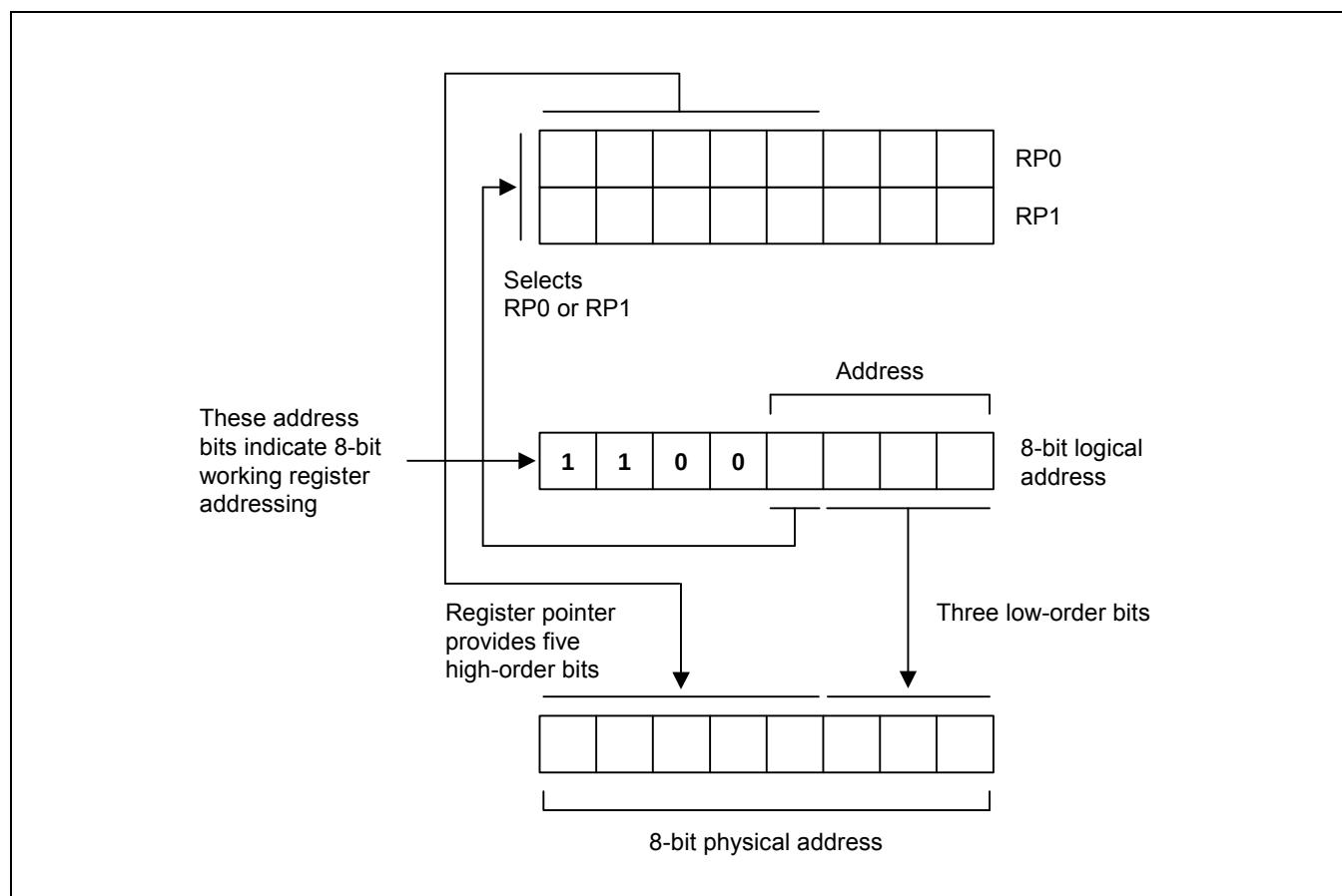
图 2-16 8 位工作寄存器寻址方式
