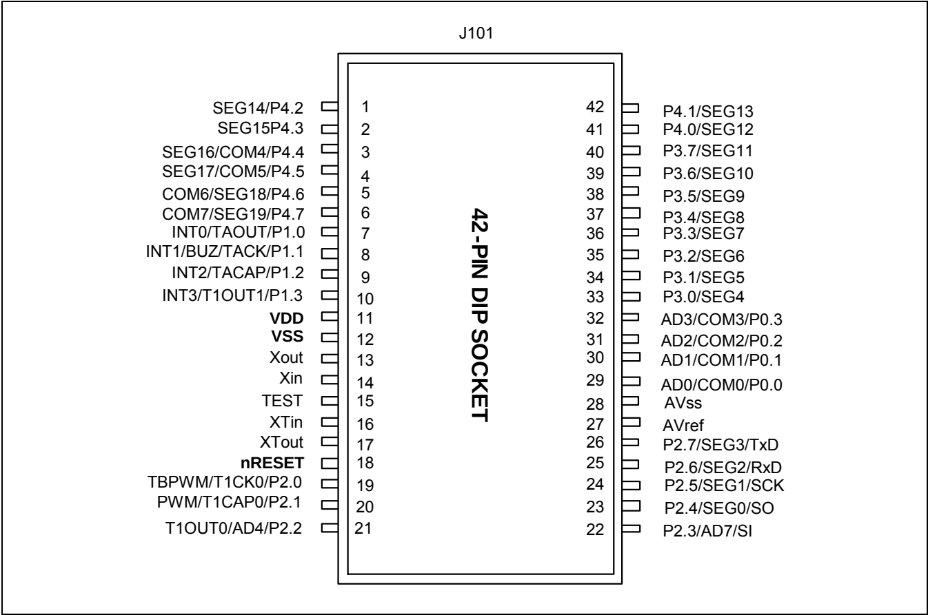
图 23-5 TB84I9的42脚接口
