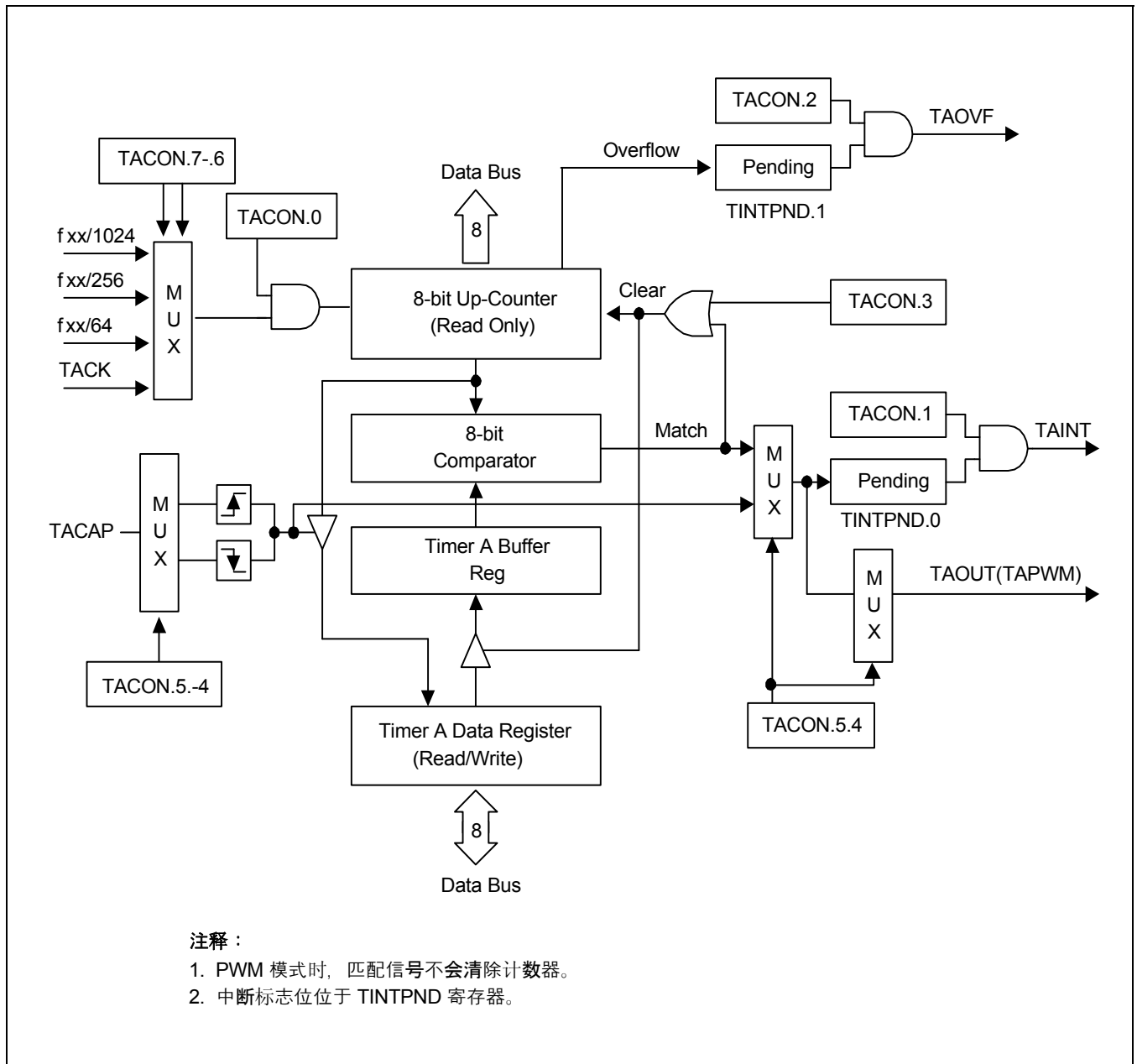
图 11-2 Timer A 功能模块框图
