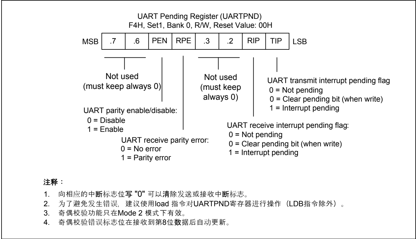
图 15-2 UART 中断标志寄存器 (UARTPND)
