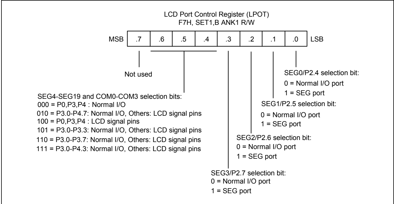
图 18-5 LCD 端口控制寄存器
