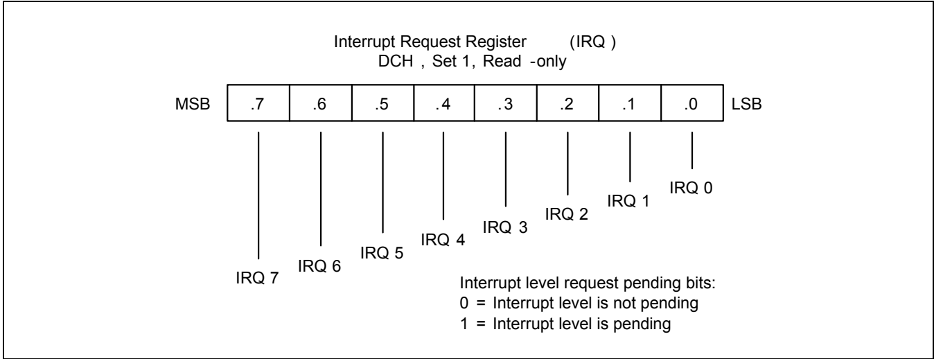
图 5-9 中断请求寄存器 (IRQ)
