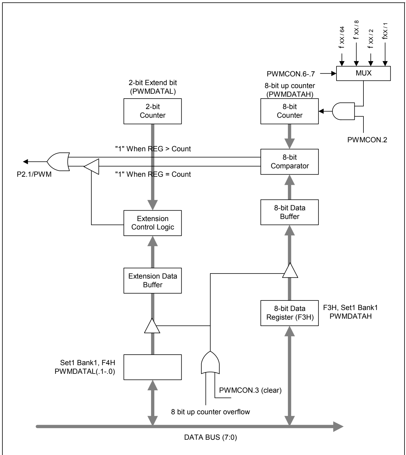
图 13-4 PWM 功能框图
