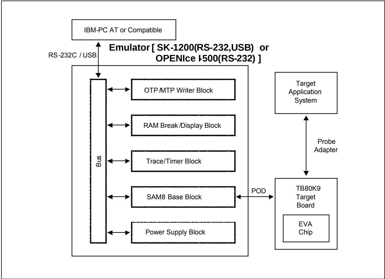
图 23-1 开发系统配置
