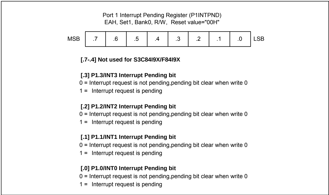
图 9-4 P1 口中断标志位寄存器
