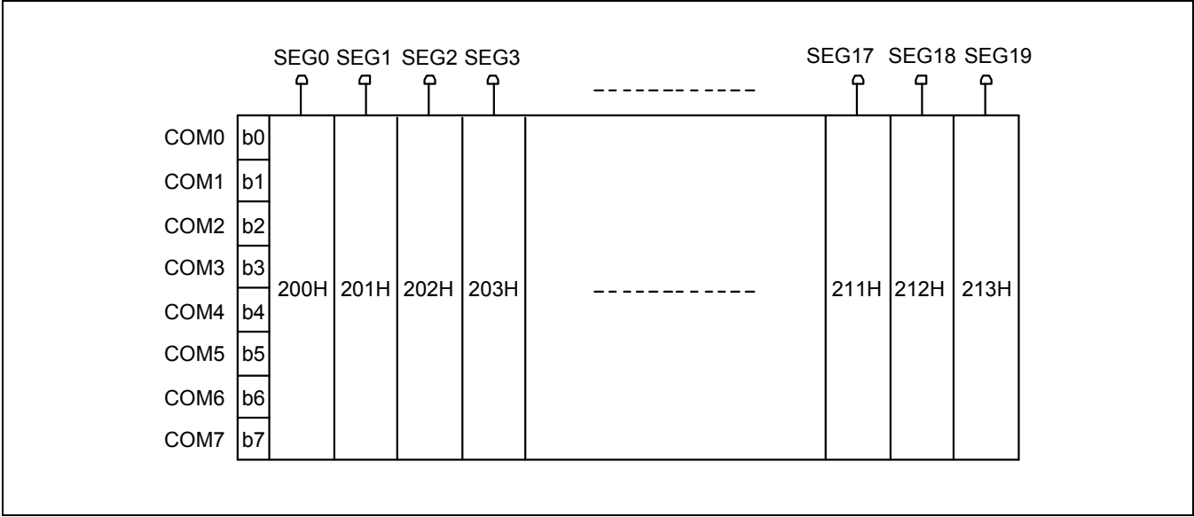
图 18-3 LCD 显示数据 RAM 结构图
