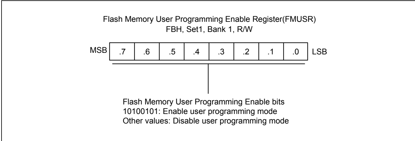
图 20-2 闪存用户编程使能寄存器 (FMUSR)
