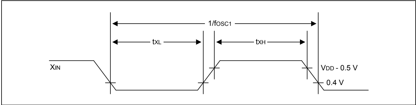
图 21-3 在X IN 的时钟时序测量值
