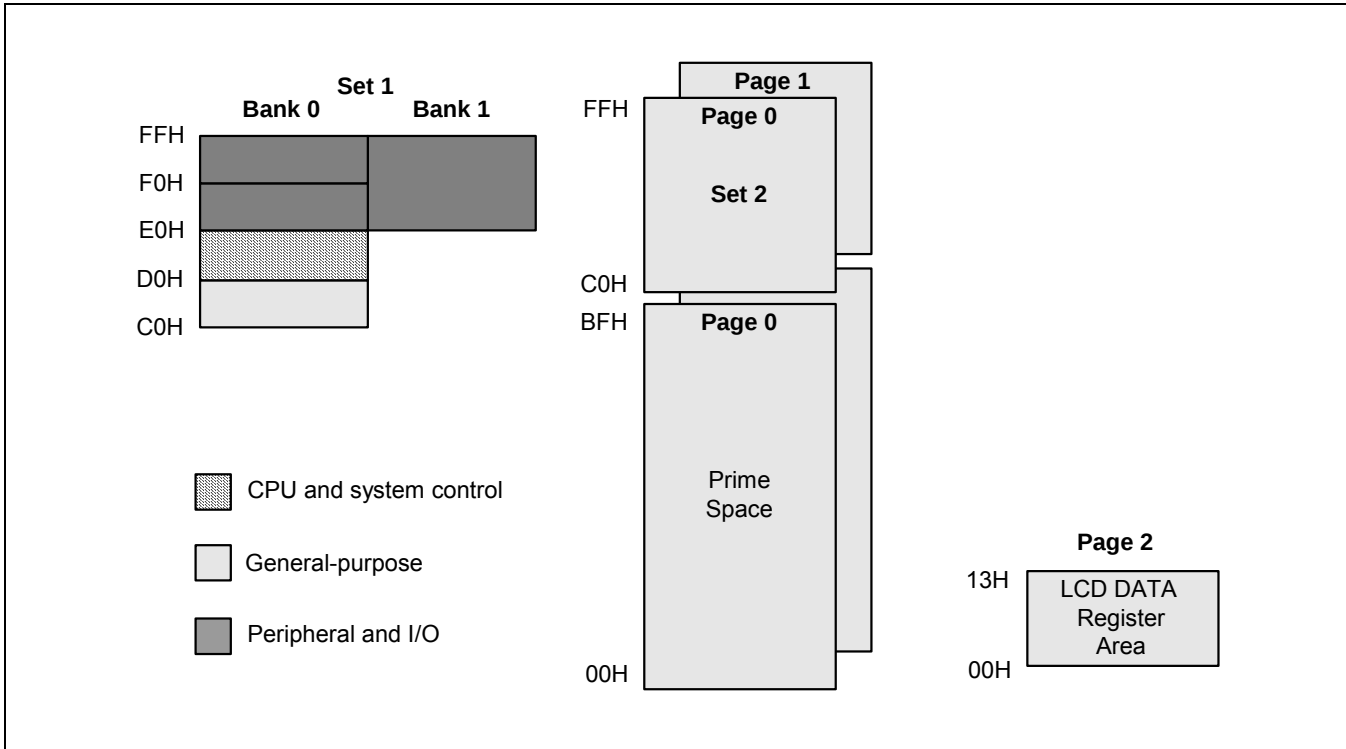
图 2-6 Set 1, Set 2, 主寄存器空间 (S3C84I9X/F84I9X)
