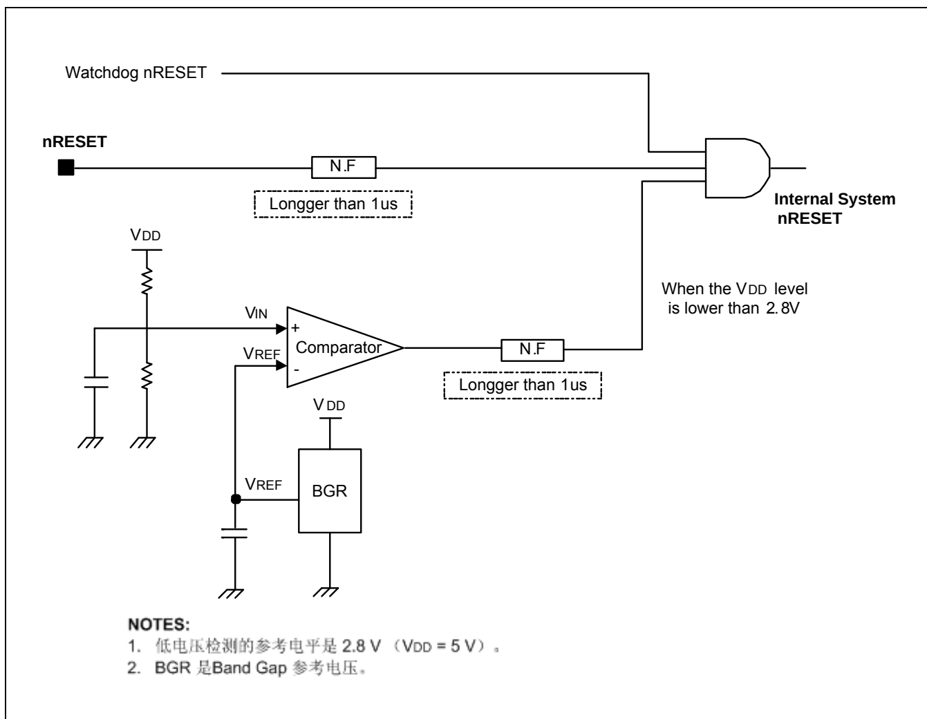
图 19-1 低压复位电路
