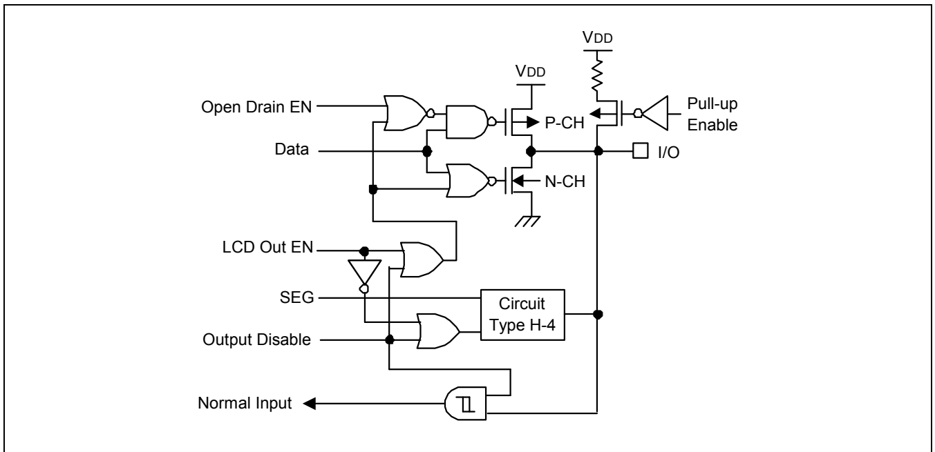
图 1-12 Pin管脚电路类型 H-17 (P3.0-P3.7, P4.0-P4.)
