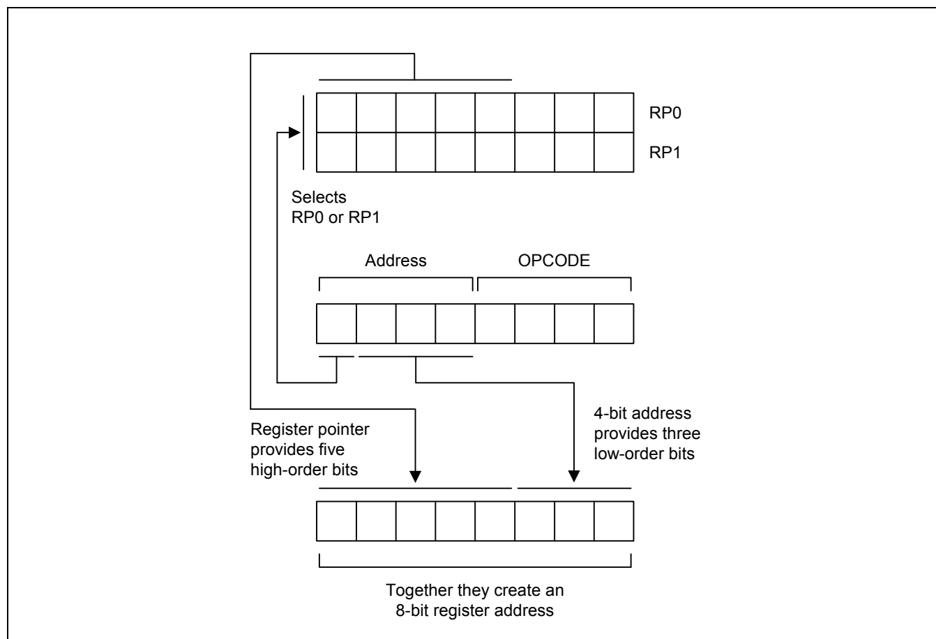
图 2-14 4 位工作寄存器寻址方式
