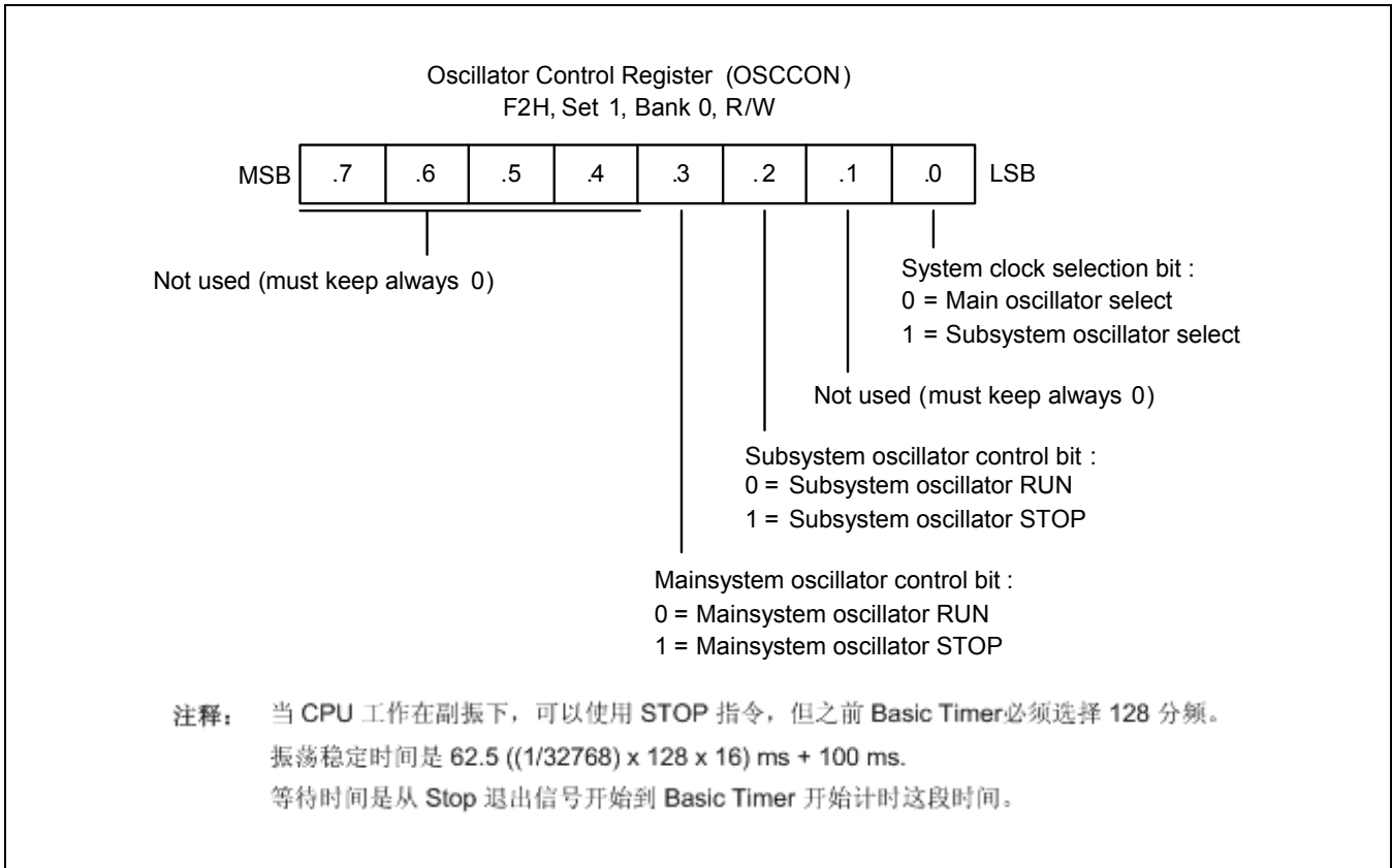
图 7-5 振荡器控制寄存器 (OSCCON)
