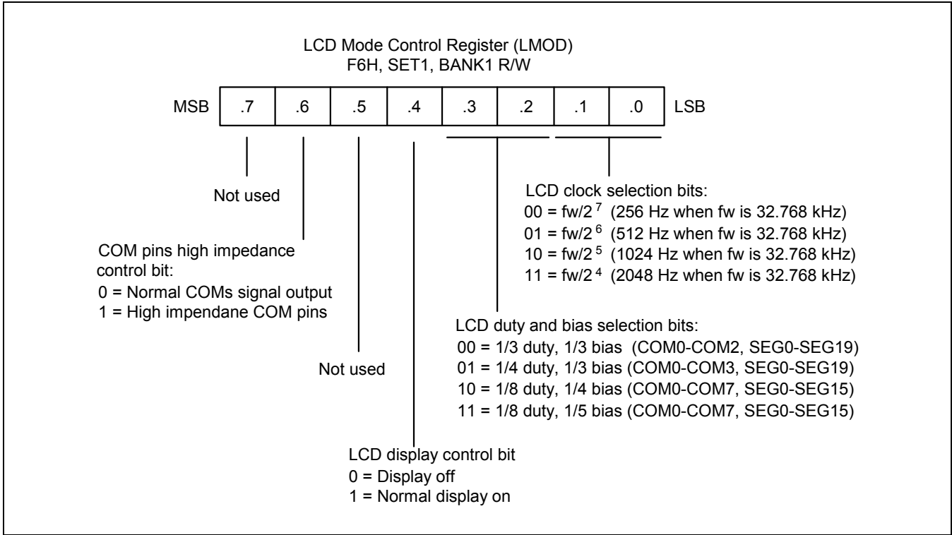
图 18-4 LCD 模式控制寄存器 (LMOD)
