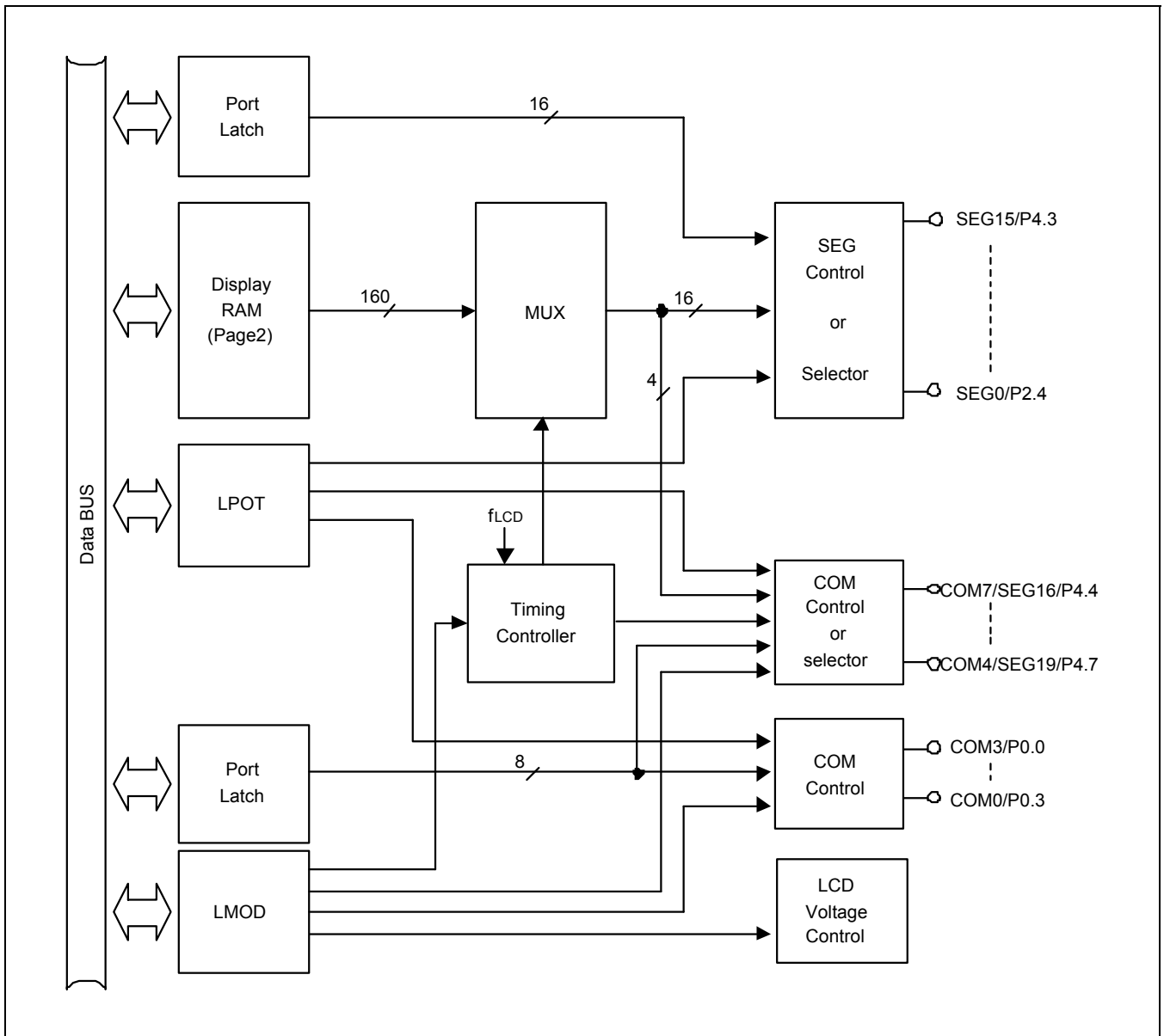
图 18-2 LCD 电路框图
