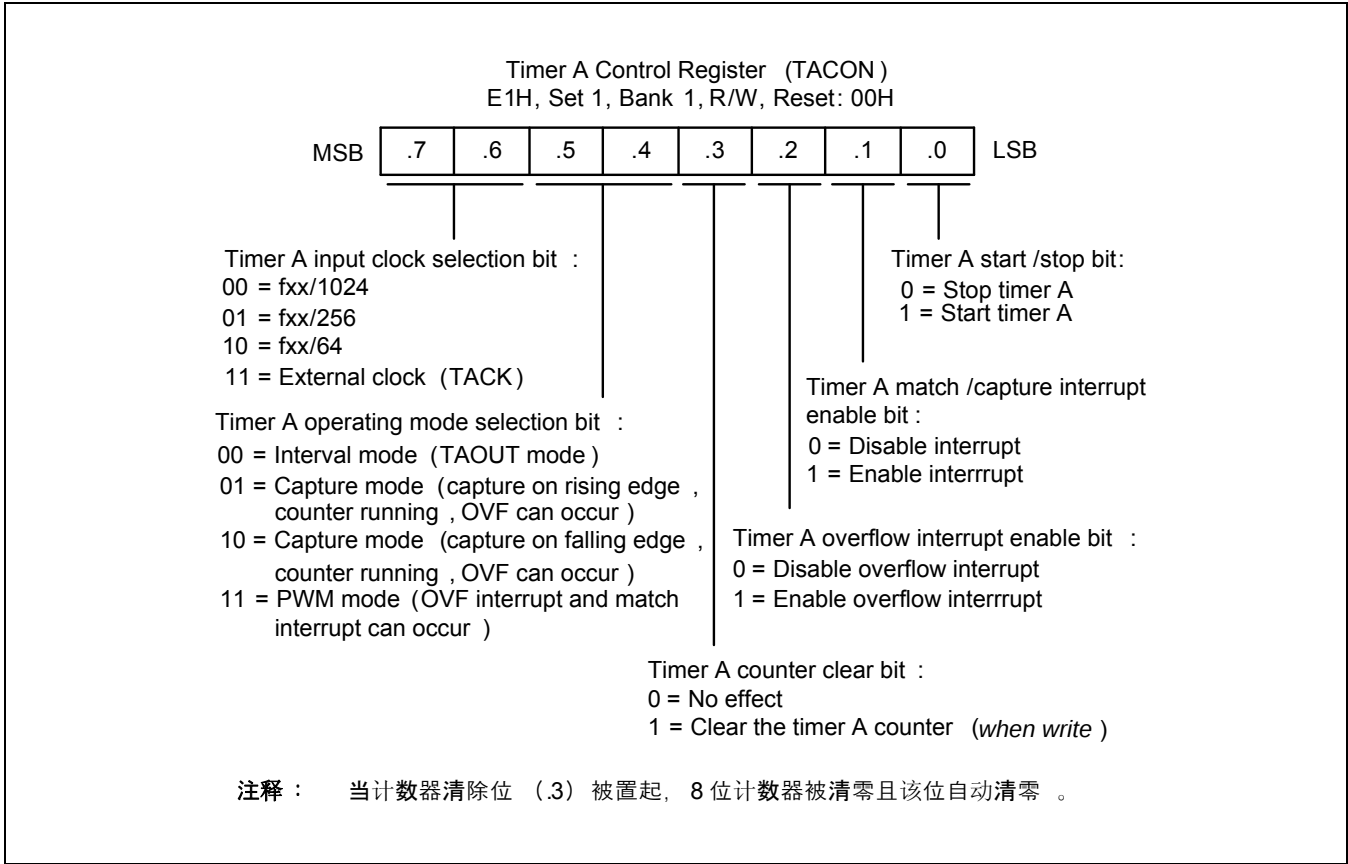
图 11-1 Timer A 控制寄存器 (TACON)
