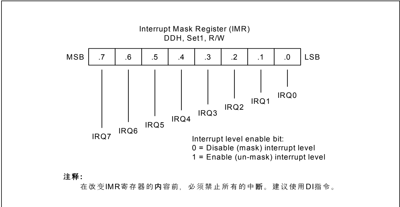
图 5-6 中断屏蔽寄存器 (IMR)
