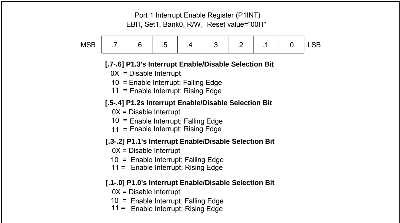
图 9-5 P1 口 中断使能寄存器 (P1INT)
