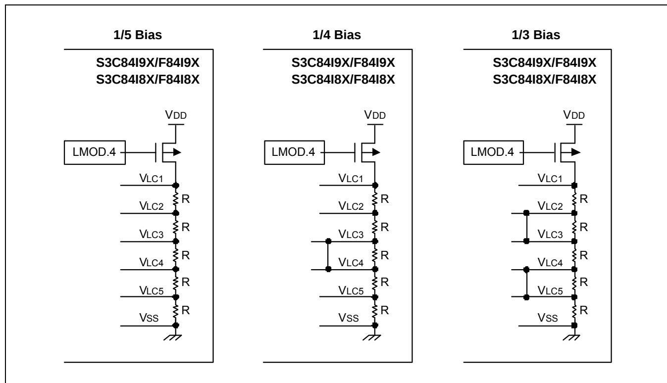
图 18-6 内部偏压电阻连接
