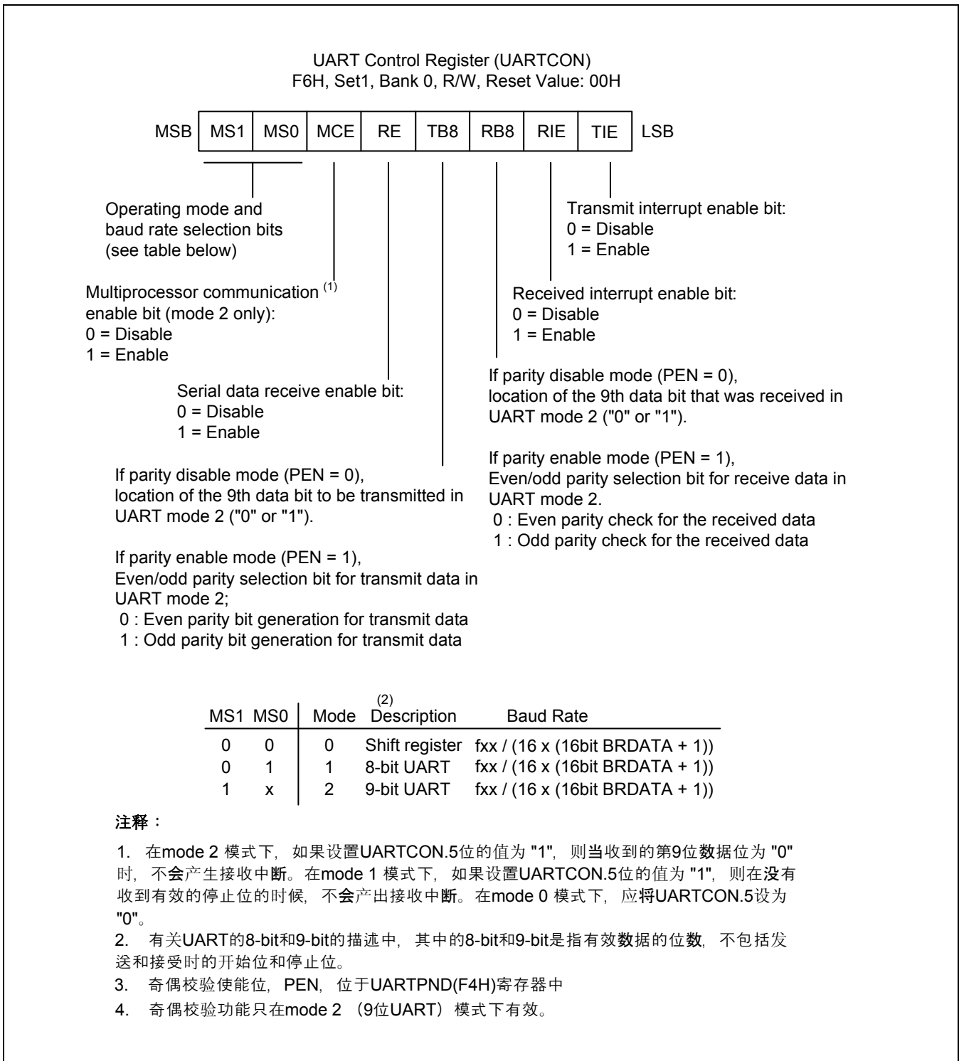
图 15-1 UART控制寄存器 (UARTCON)
