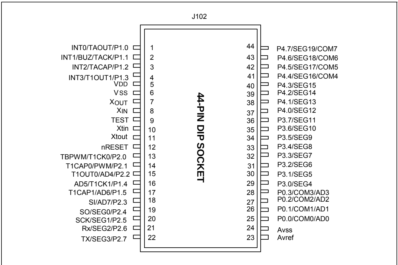
图 23-4 TB84I9的44脚接口
