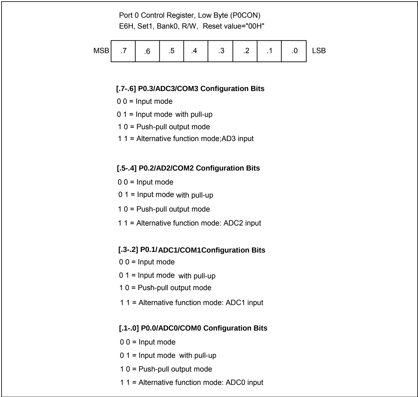
图 9-1 P0 口低字节控制寄存器 (P0CON)
