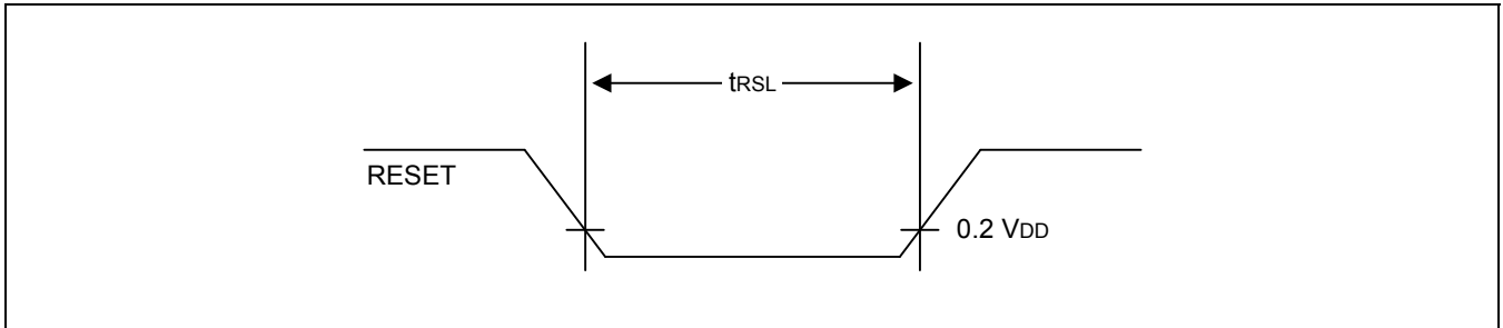
图 21-2 nRESET 输入时序
