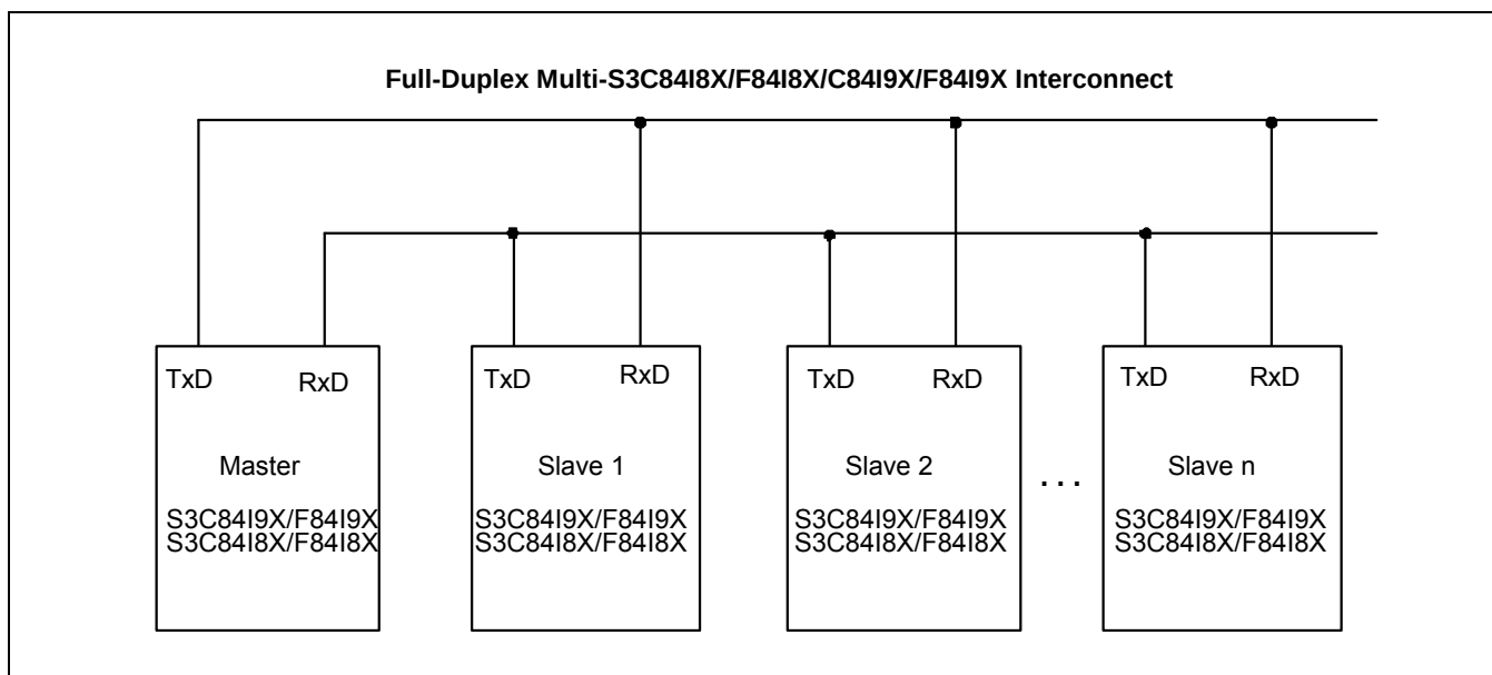
图 15-9 多节点串行通讯连接示例
