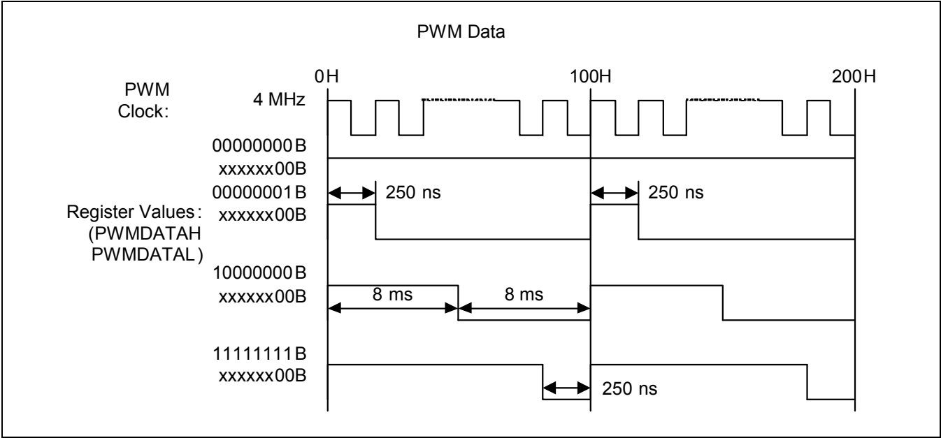
图 13-1 PWM基本波形 (8位)
