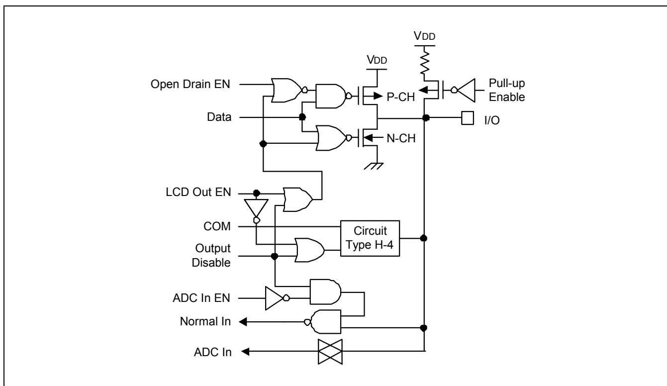
图 1-11 管脚电路类型 H-16 (P0.0-P0.3)
