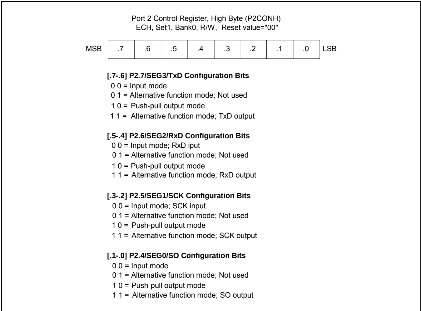
图 9-6 P2 口 高字节控制寄存器 (P2CONH)
