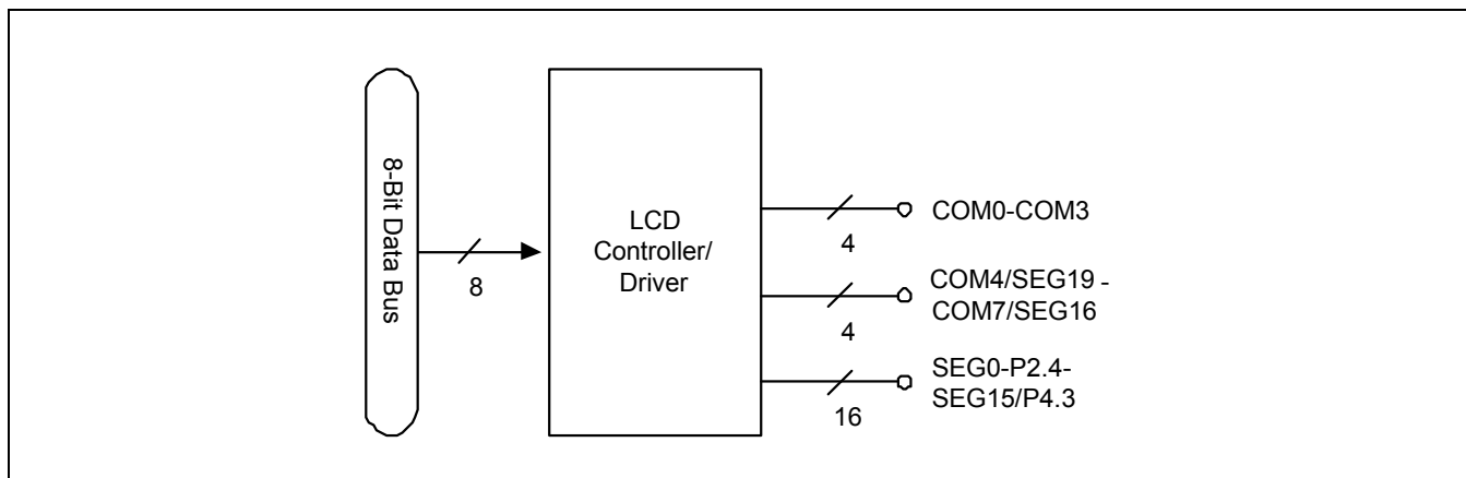
图 18-1 LCD 功能方框图
