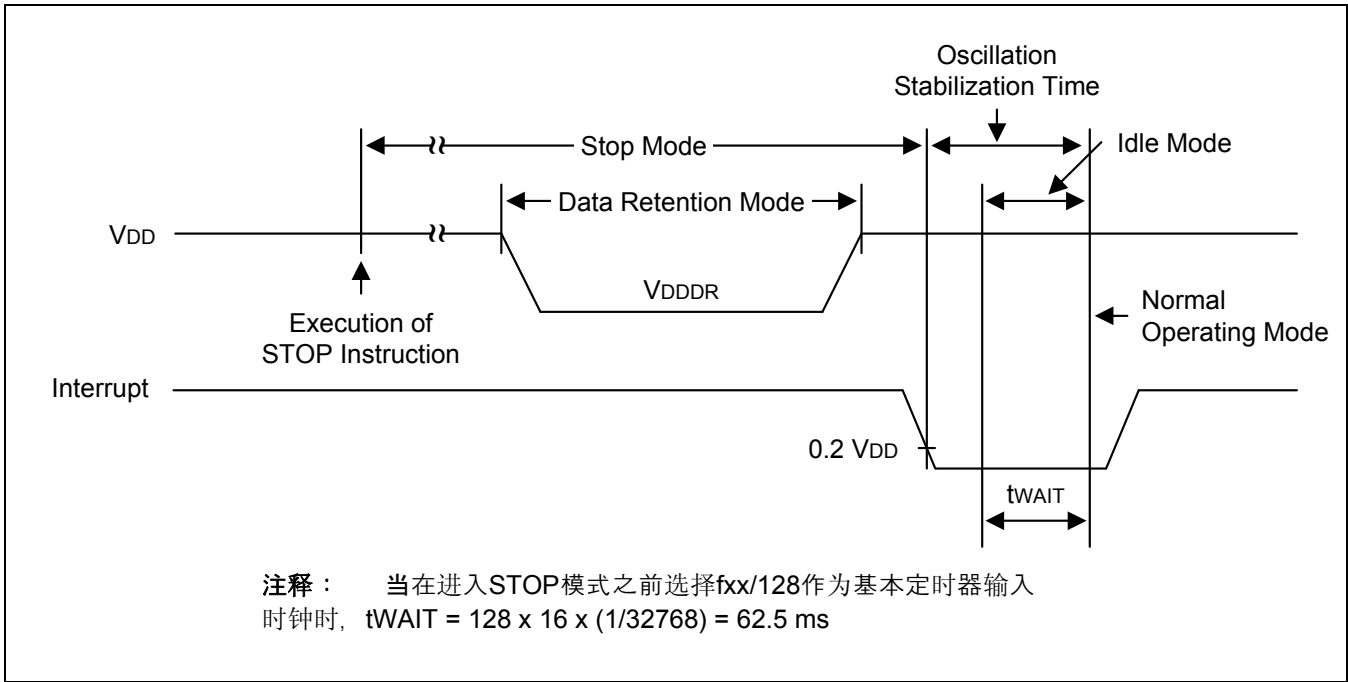
图 21-6 中断使系统退出 STOP 模式(子系统)时序图
