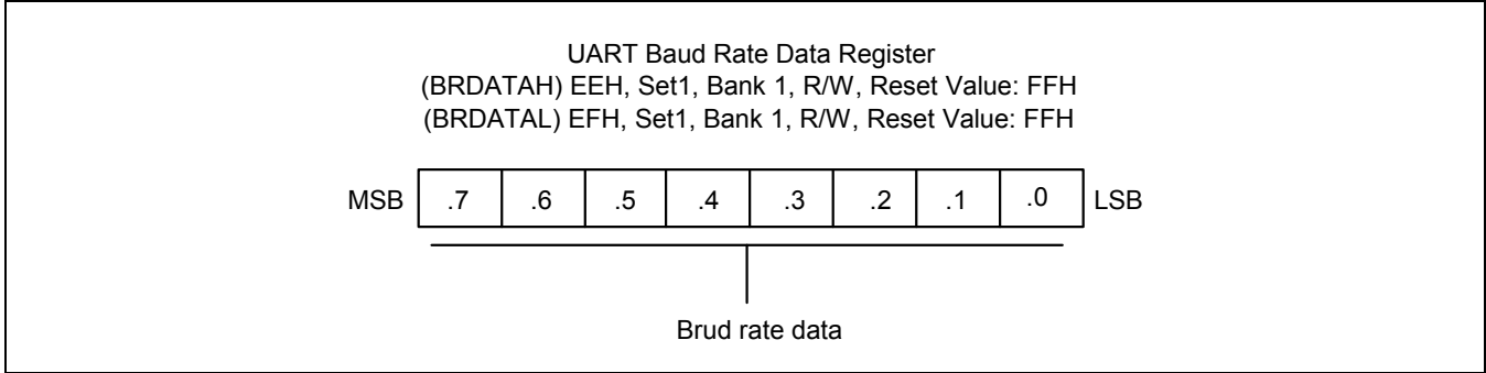
图 15-4 UART 波特率数据寄存器 (BRDATAH, BRDATAL)
