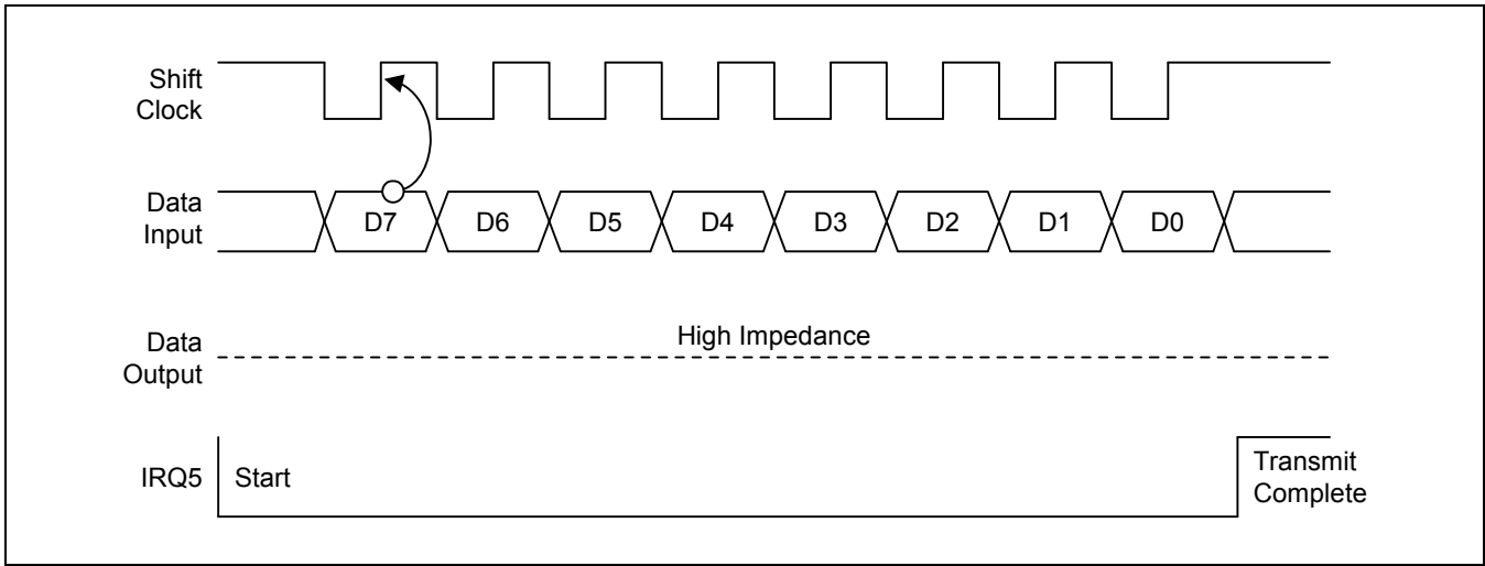
图 14-6 SIO 仅接收模式时序图
