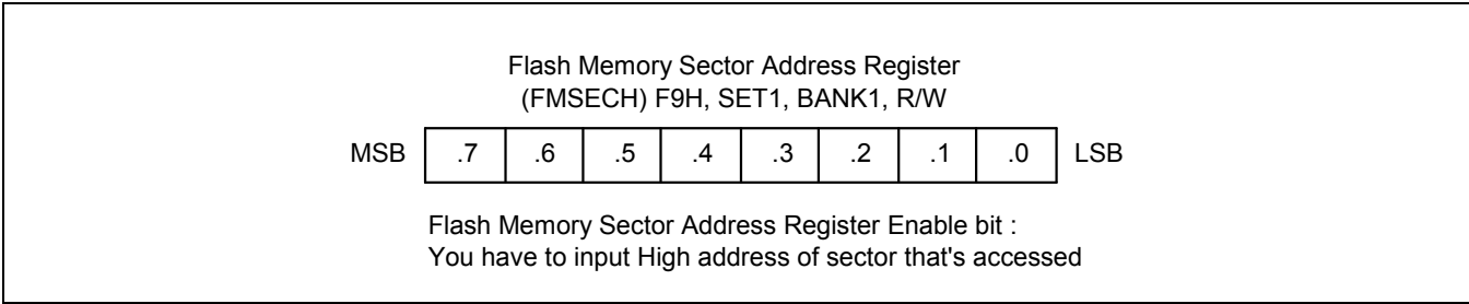
图 20-4 闪存扇区地址寄存器高字节 (FMSECH)
