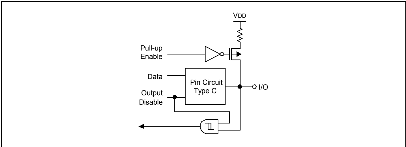
图 1-6 管脚电路类型D
