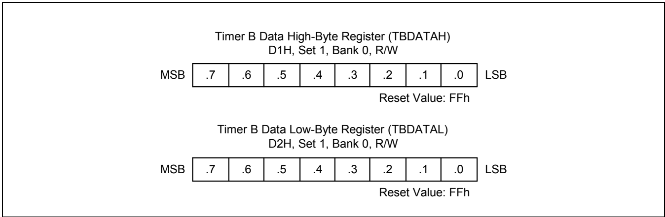
图 11-5 Timer B 数据寄存器 (TBDATAH, TBDATAL)
