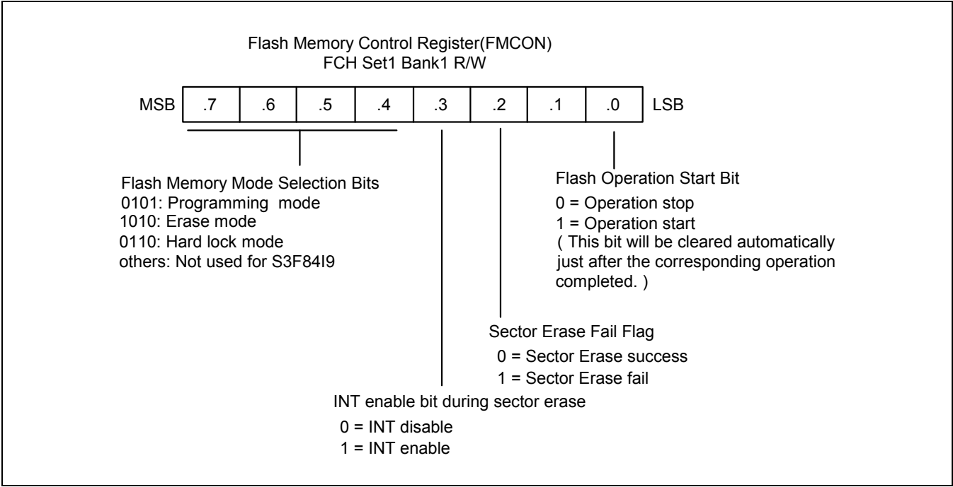
图 20-1 闪存控制寄存器 (FMCON)
