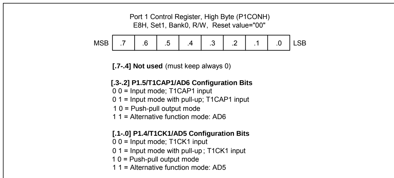
图 9-2 P1 口高字节控制寄存器 (P1CONH)
