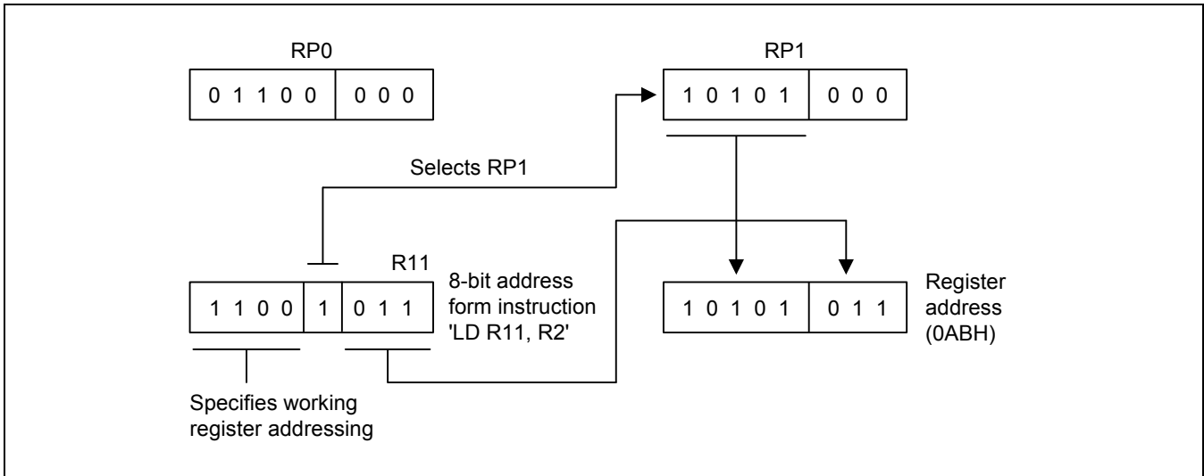
图 2-17 8 位工作寄存器寻址实例
