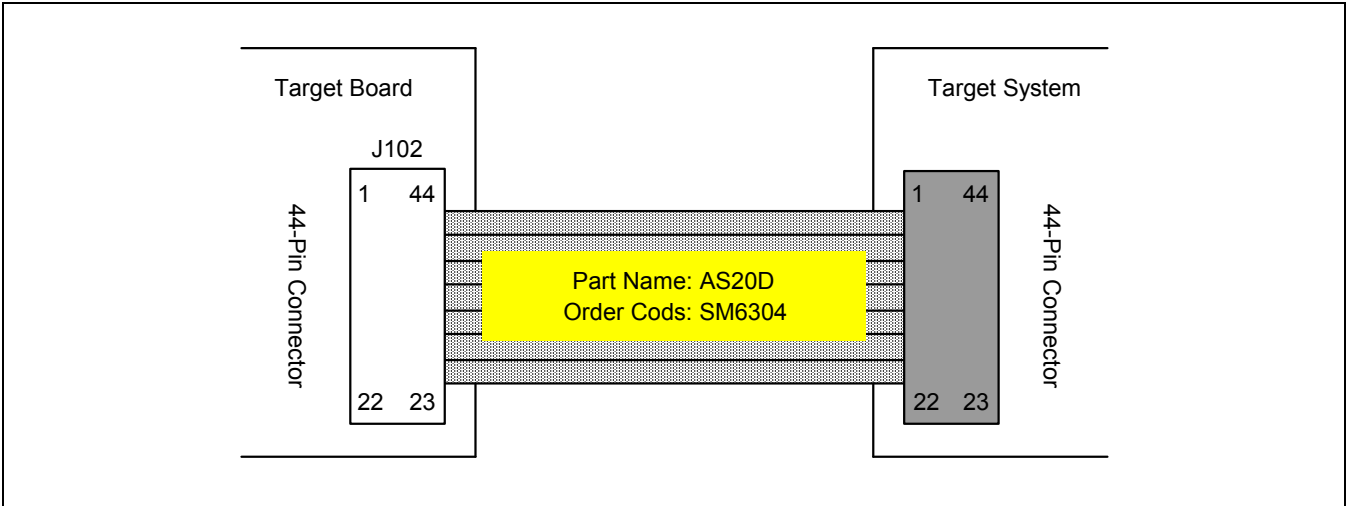
图 23-6 44 脚封装的 TB84I9 适配器数据线
