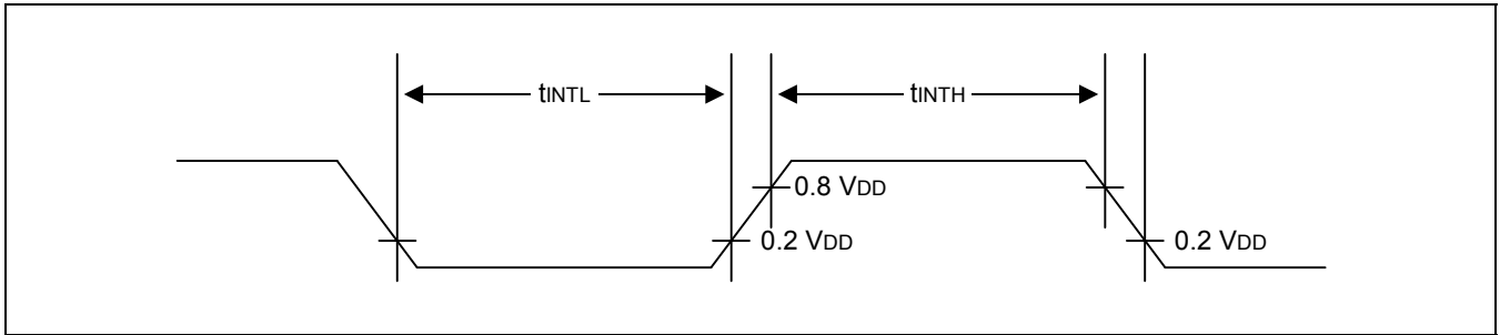
图 21-1 外部中断输入时序 (Ports 2)
