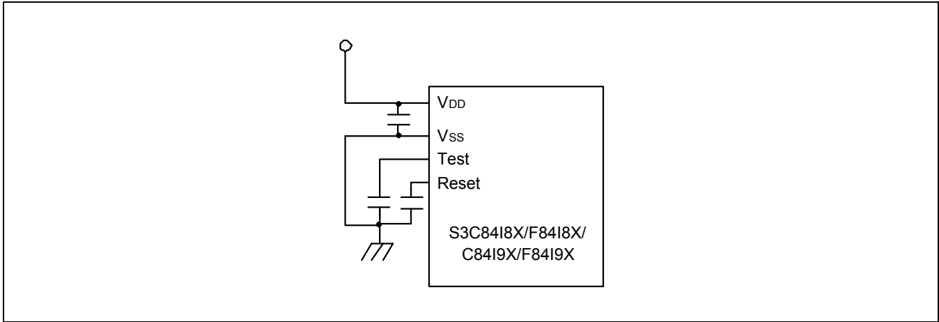
图 21-9 改进 EFT 特性的电路图
