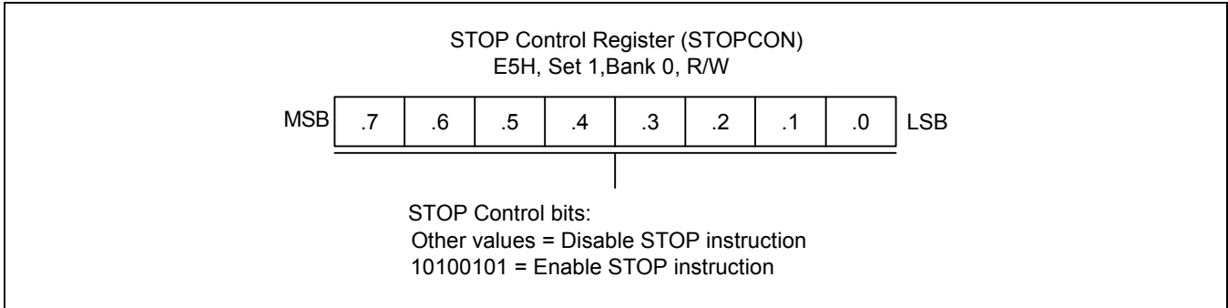
图 7-6 STOP 控制寄存器 (STOPCON)
