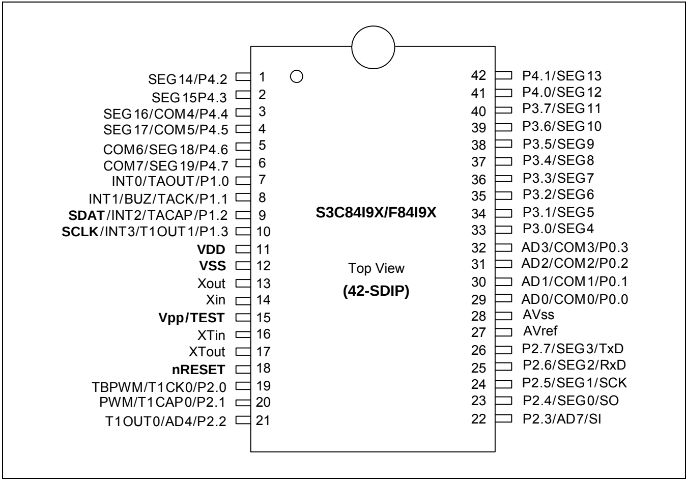
图 1-3 S3C84I9X/F84I9X管脚分布图 (42- SDIP)
