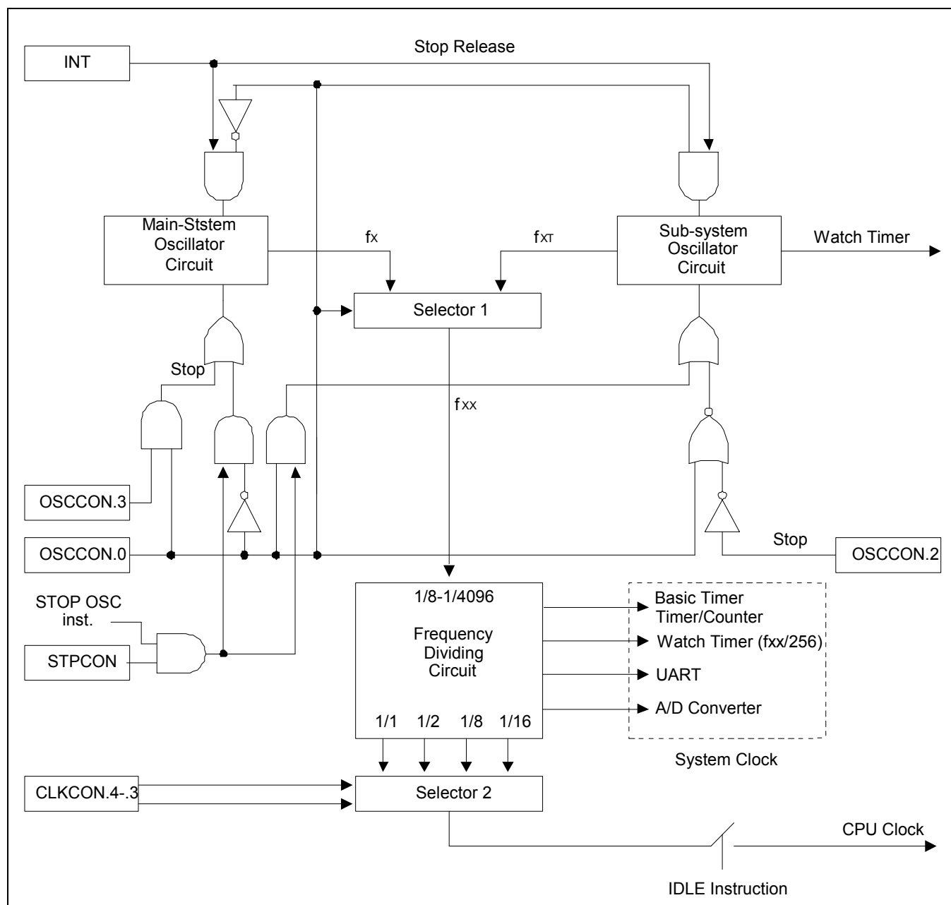
图 7-3 系统时钟电路原理图
