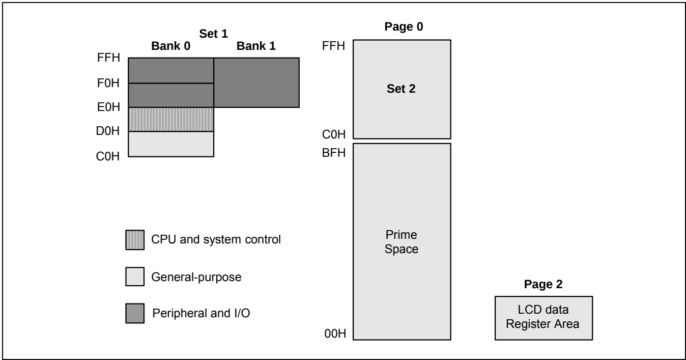
图 2-7 Set 1, Set 2, 主寄存器空间 (S3C84I8X/F84I8X)
