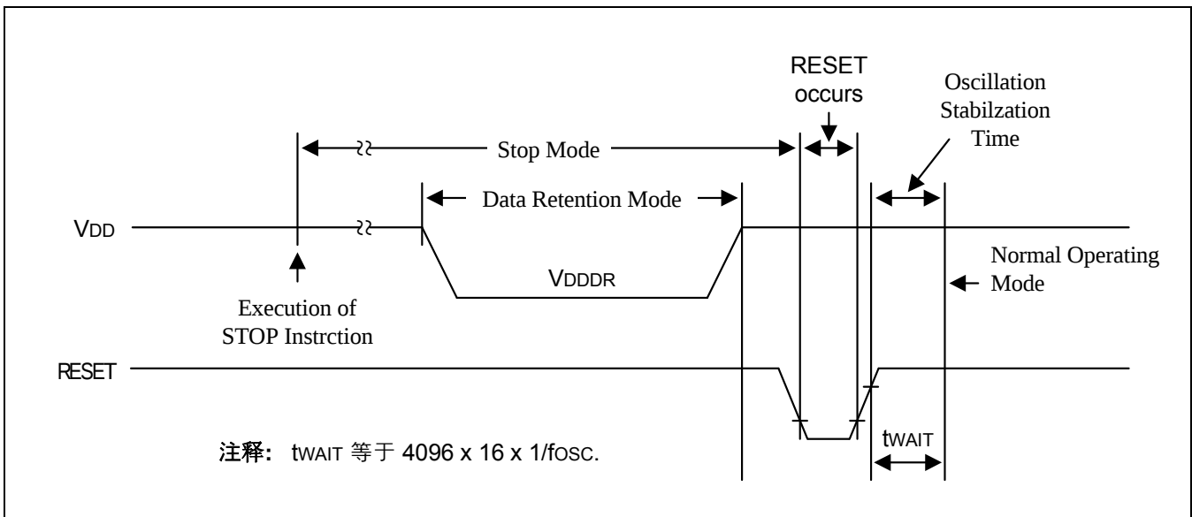
图 21-4 复位使系统退出 STOP 模式时序图
