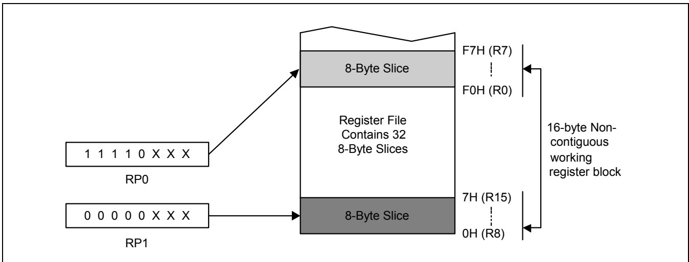
图 2-10 非相邻的 16 字节工作寄存器块
