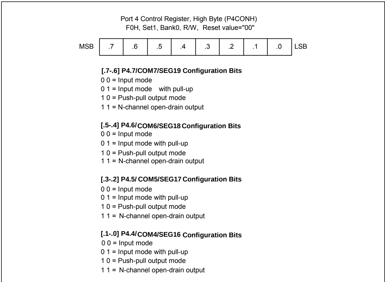
图 9-11 P4 口高字节控制寄存器 (P4CONH)
