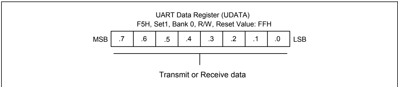
图 15-3 UART 数据寄存器 (UDATA)
