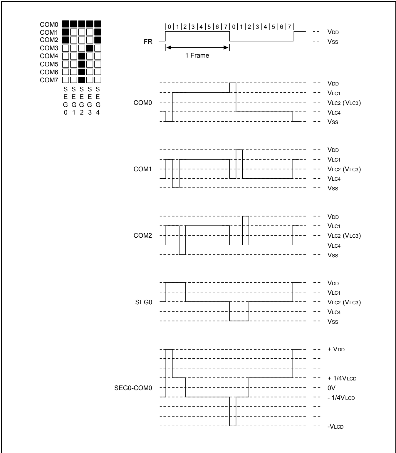
图 18-7 LCD 信号波形 (1/8 占空比, 1/4 偏压比)
