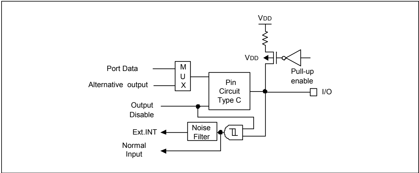
图 1-7 管脚电路类型D-5 (P1.0-P1.3)
