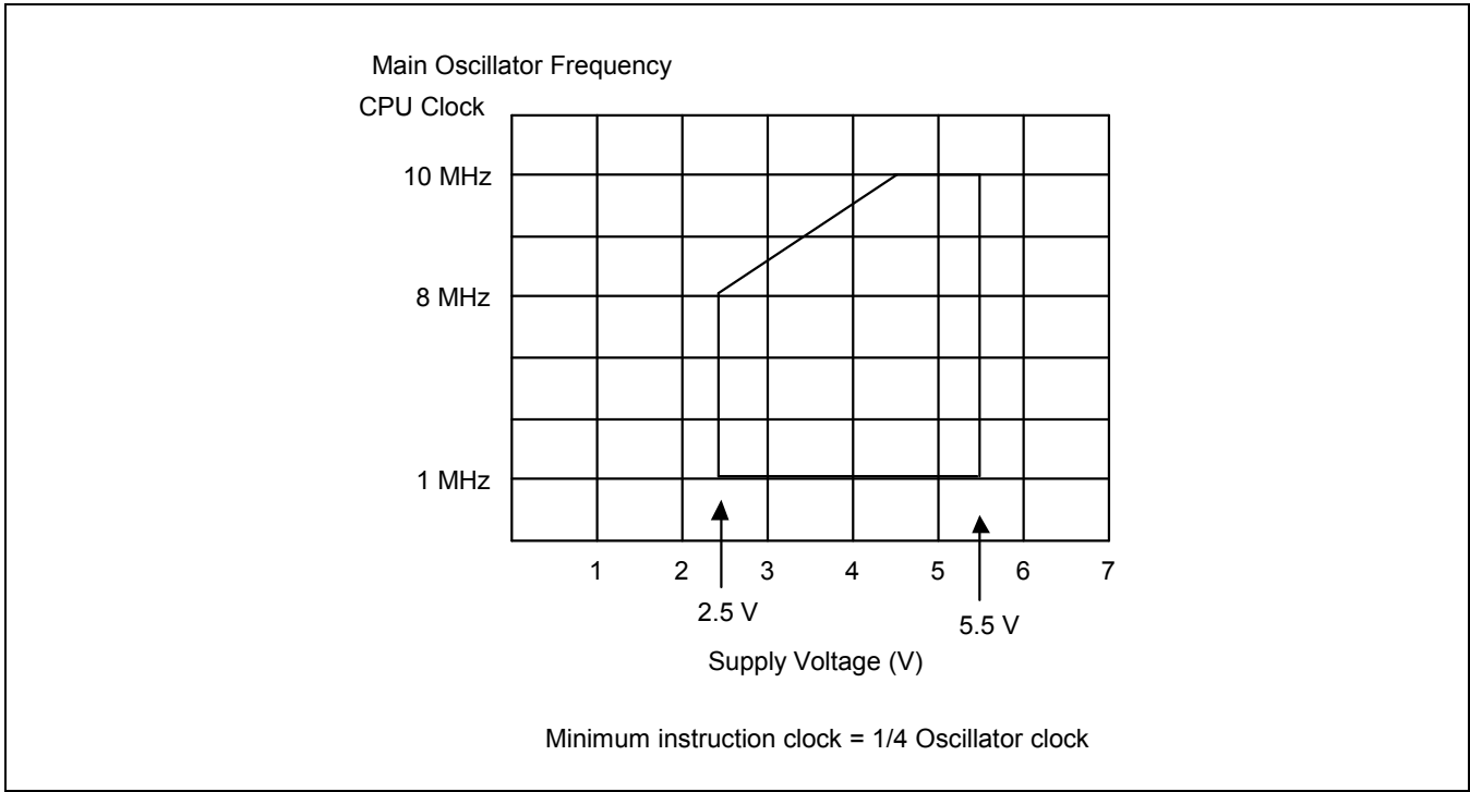
图 21-8 工作电压范围
