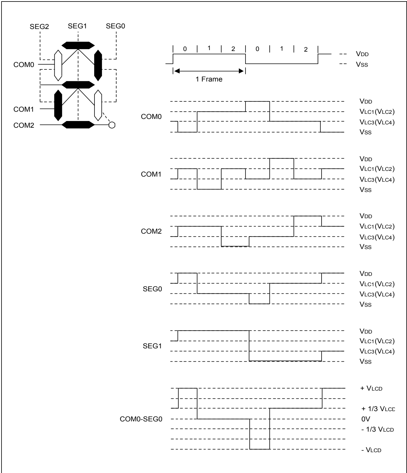
图 18-9 LCD 信号波形 (1/3 占空比, 1/3 偏压比)
