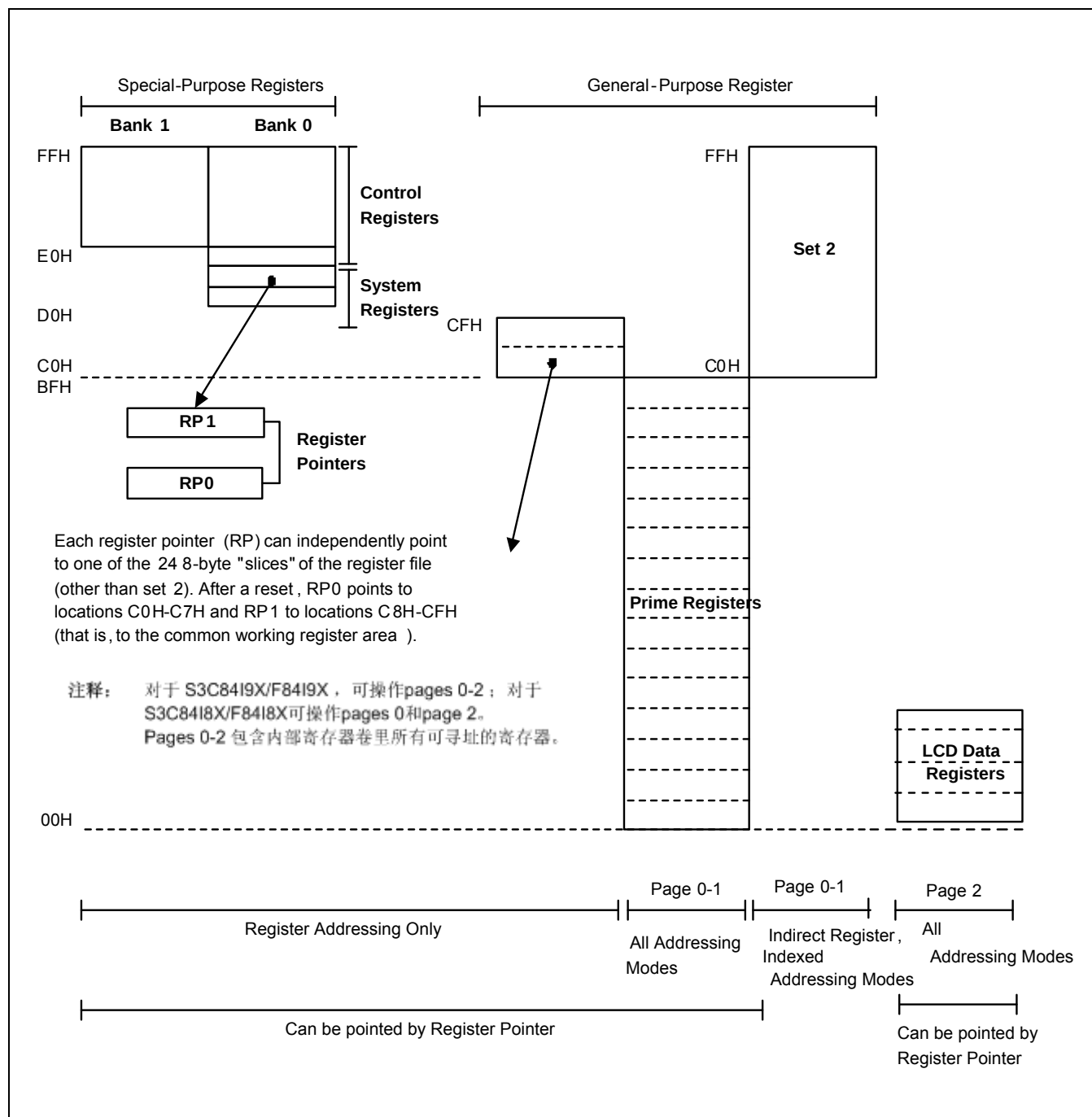
图 2-12 寄存器卷寻址模式
