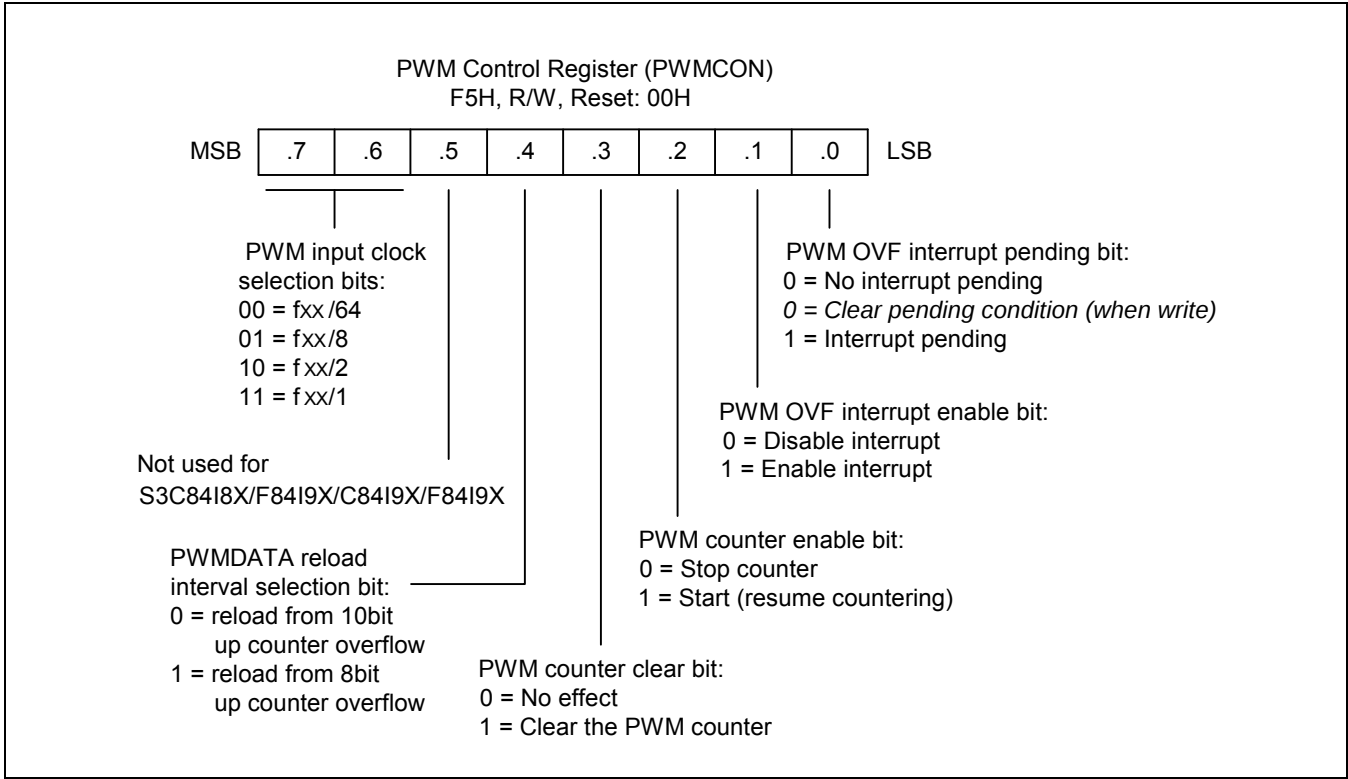
图 13-3 PWM 控制寄存器 (PWMCON)
