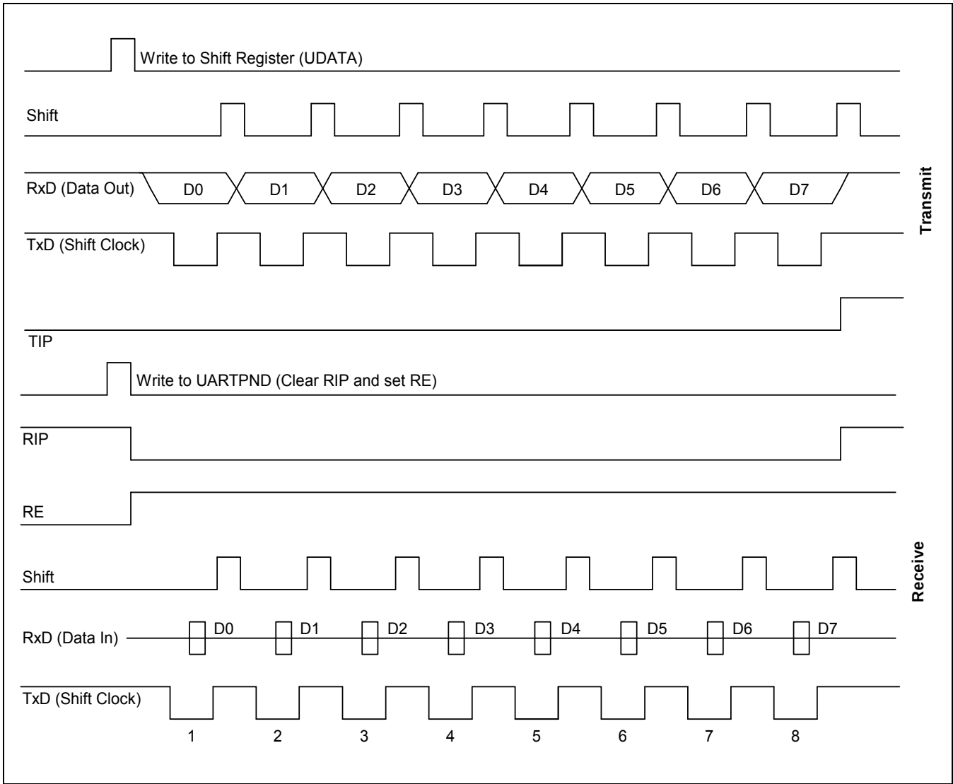
图 15-6 UART Mode 0 模式运行时序图
