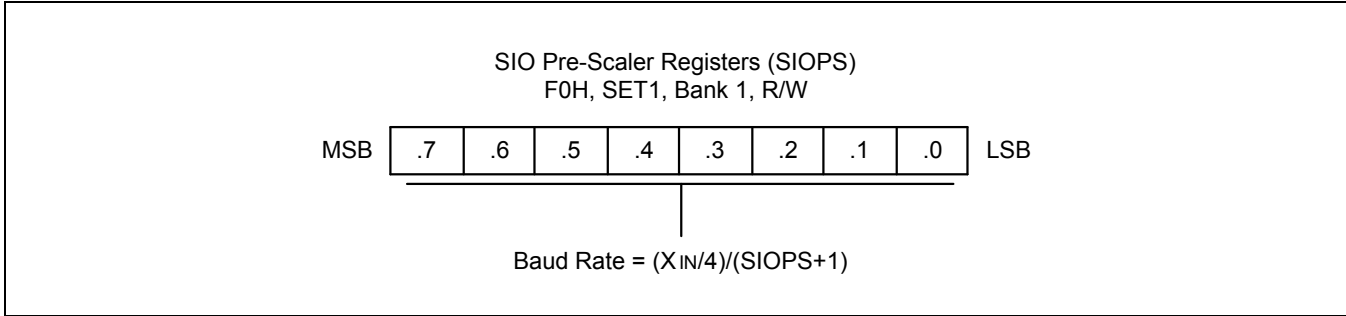
图 14-2 SIO 预分频寄存器 (SIOPS)
