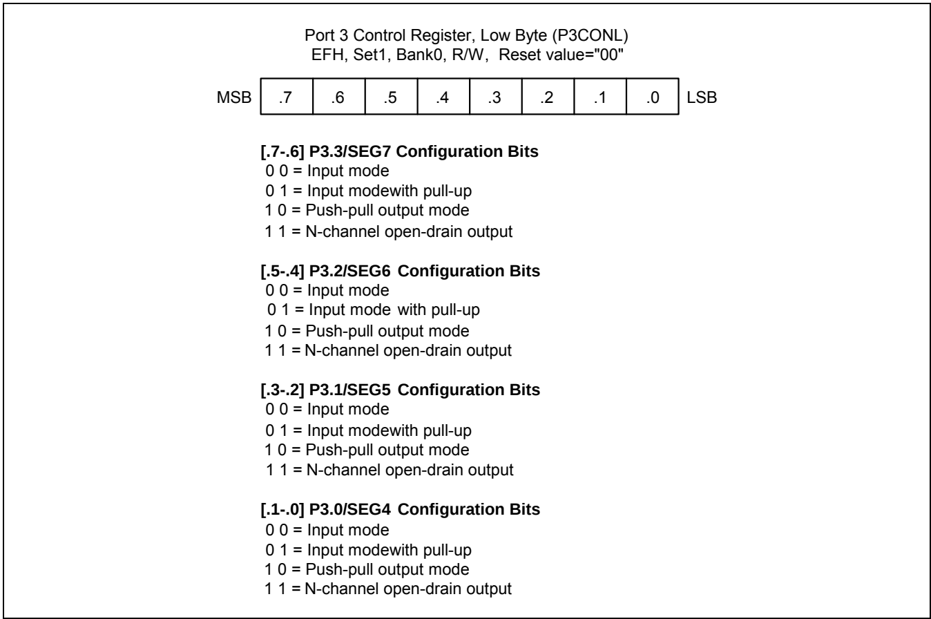
图 9-10 P3 口低字节控制寄存器 (P3CONL)
