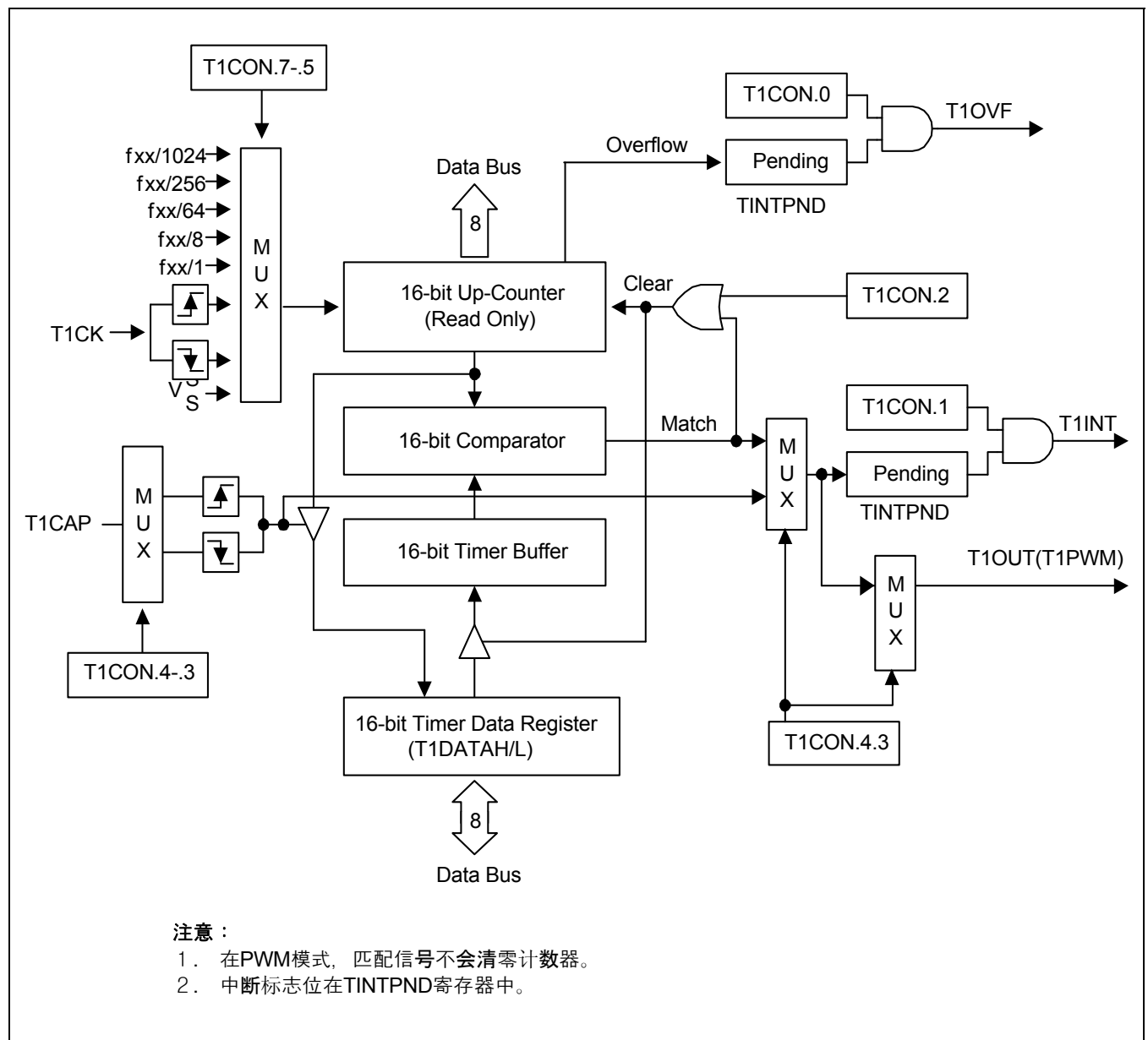
图 12-3 Timer 1(0,1) 功能框图
