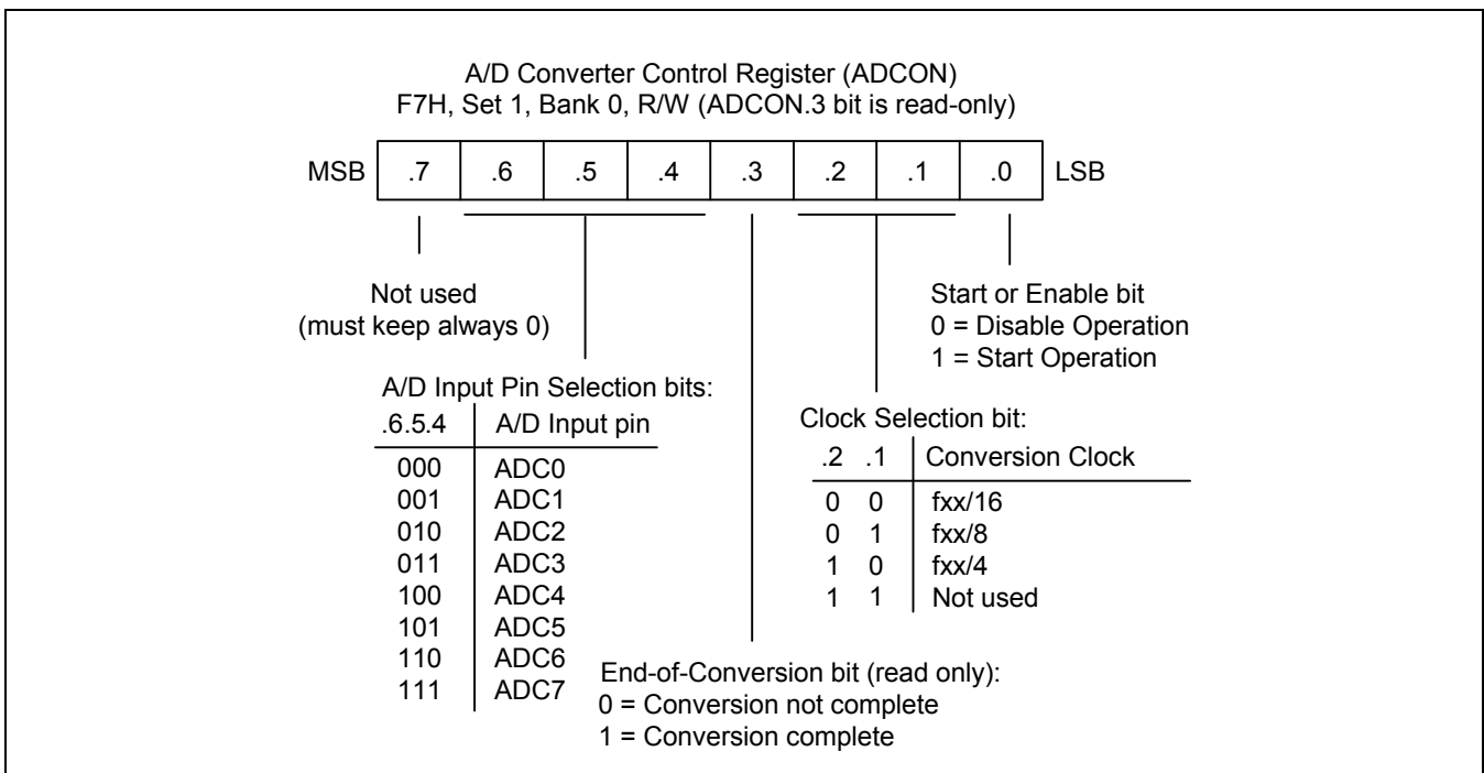
图 16-1 A/D 转换控制寄存器 (ADCON)
