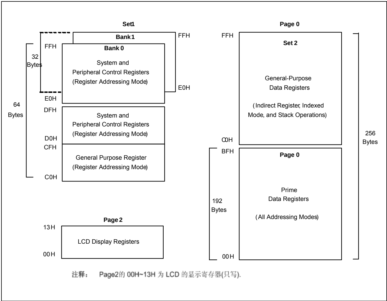
图 2-4 S3F84I8X/C84I8X 内部寄存器卷的地址空间
