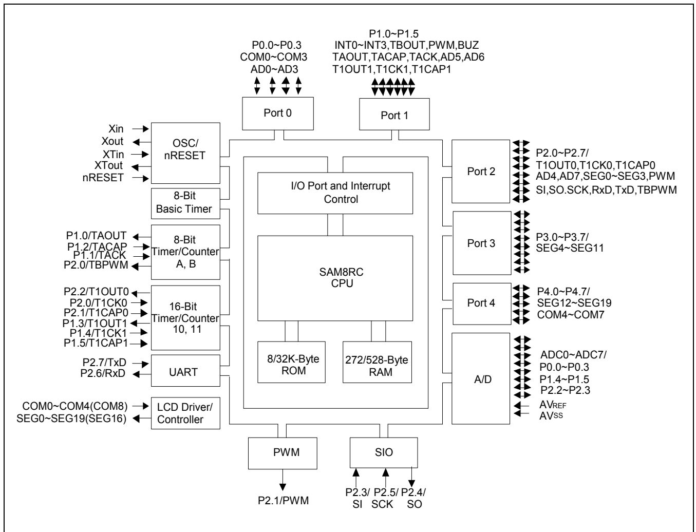
图 1-1 S3C84I8/F84I8/C84I9/F84I9 系统框图
