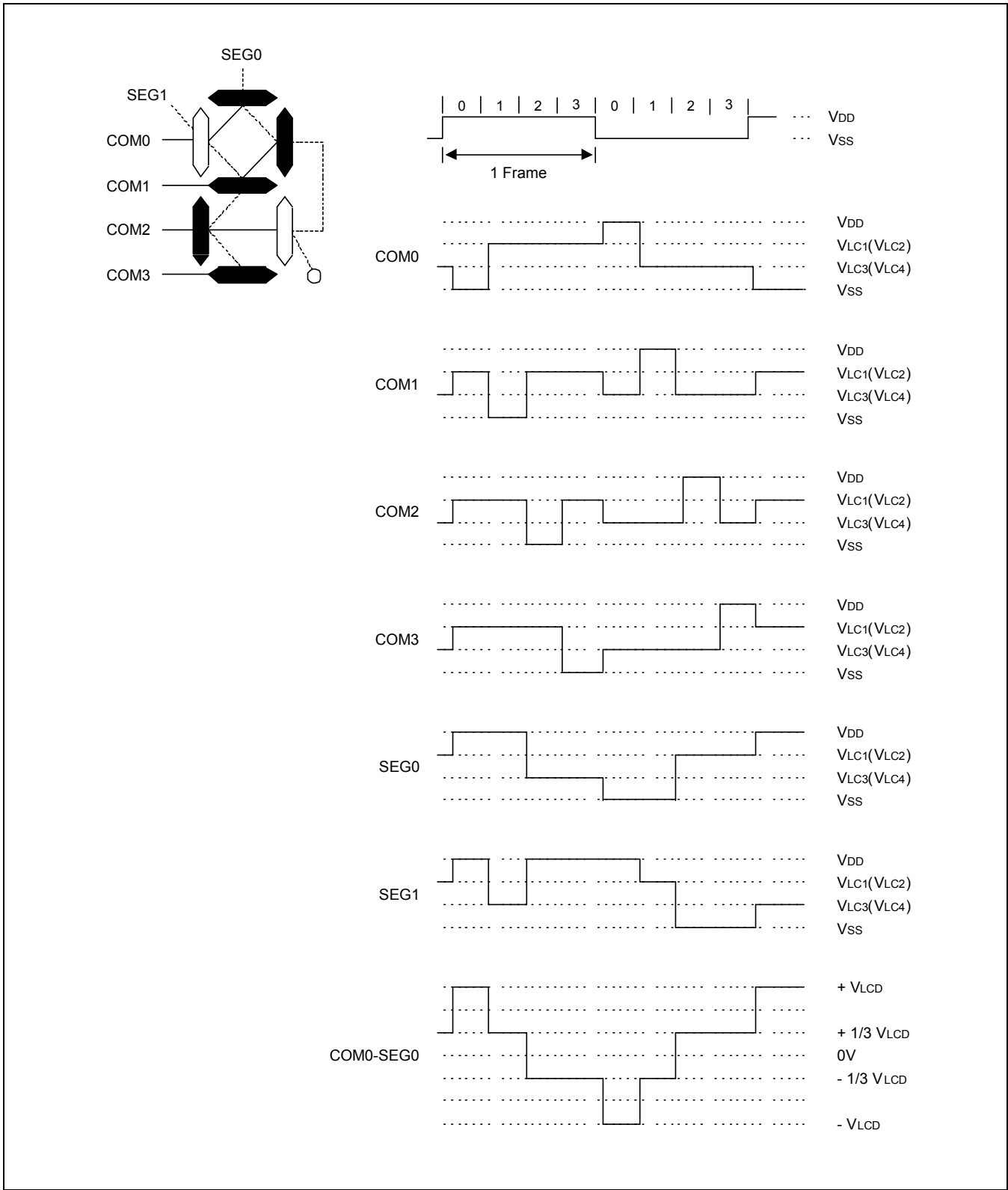
图 18-8 LCD 信号波形 (1/4占空比, 1/3 偏压比)
