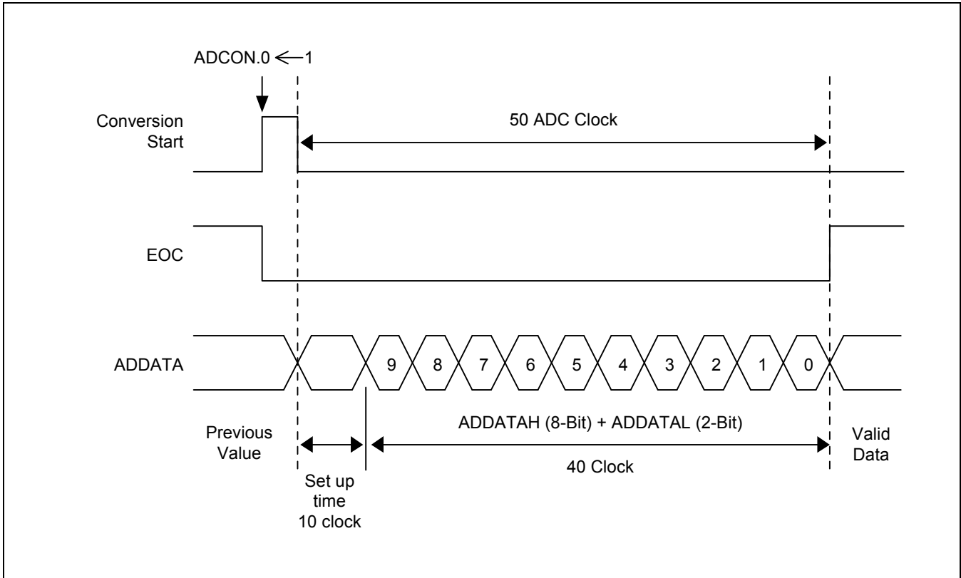
图 16-4 A/D 转换时序图
