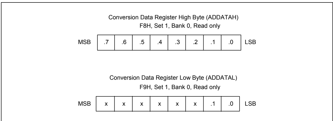
图 16-2 A/D 转换数据寄存器 (ADDATAH, ADDATAL)
