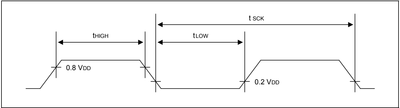
图 21-7 UART时序特性波形
