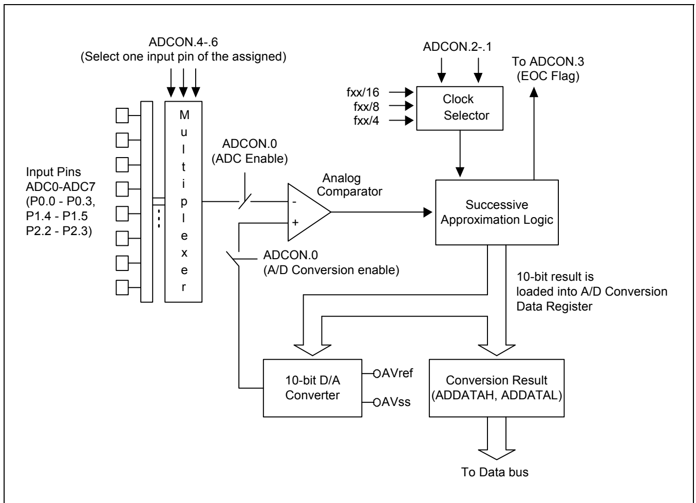
图 16-3 A/D 转换器电路图
