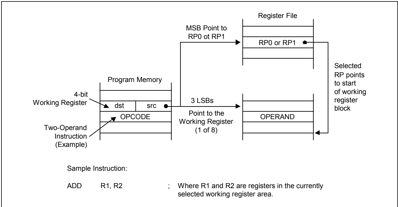
图 3-2 工作寄存器寻址模式
