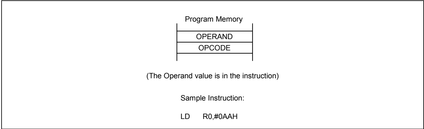
图 3-14 立即数寻址模式
