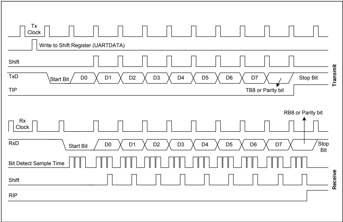
图 15-8 UART Mode 2 模式运行时序图
