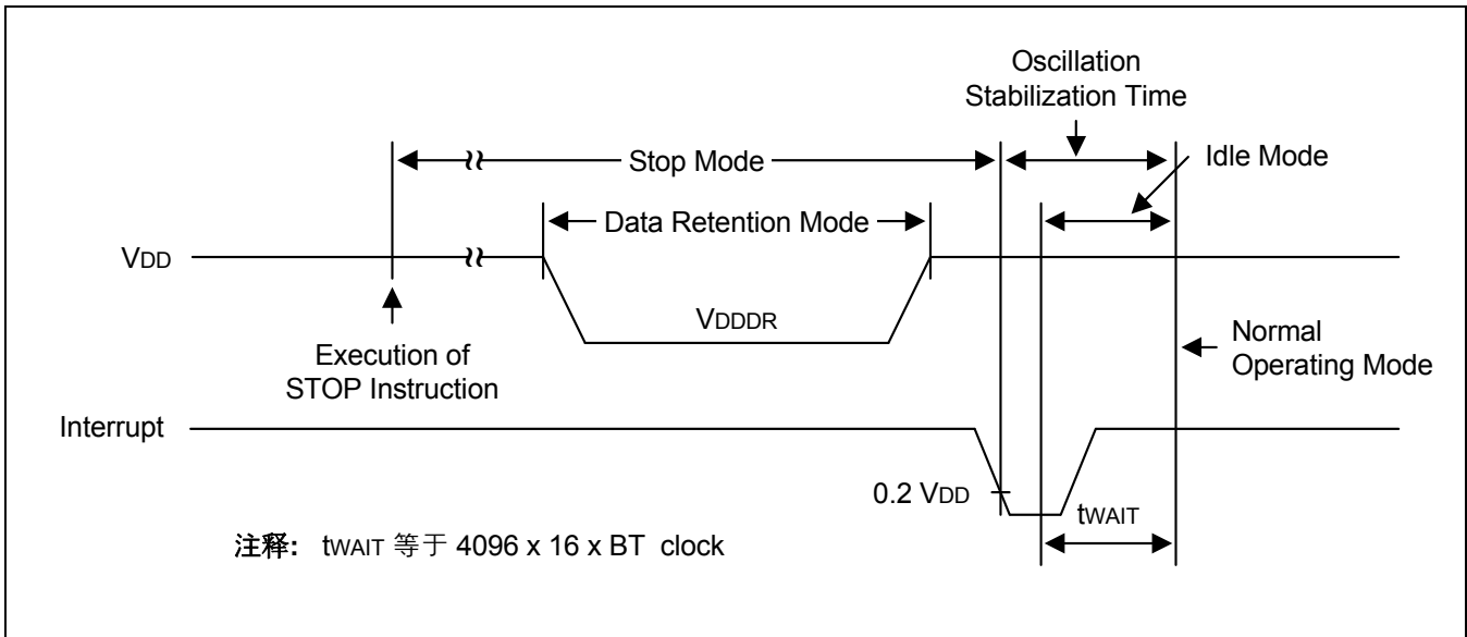
图 21-5 中断使系统退出 STOP 模式(主系统)时序图
