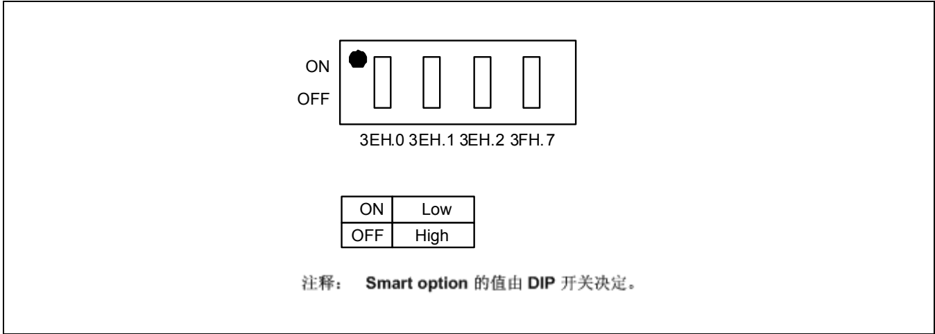
图 23-3 Smart Option 的DIP开关
