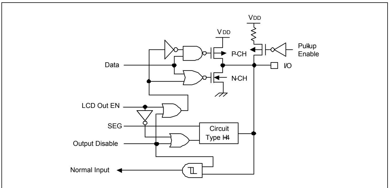
图 1-13 管脚电路类型 H-18 (2.4-P2.7)
