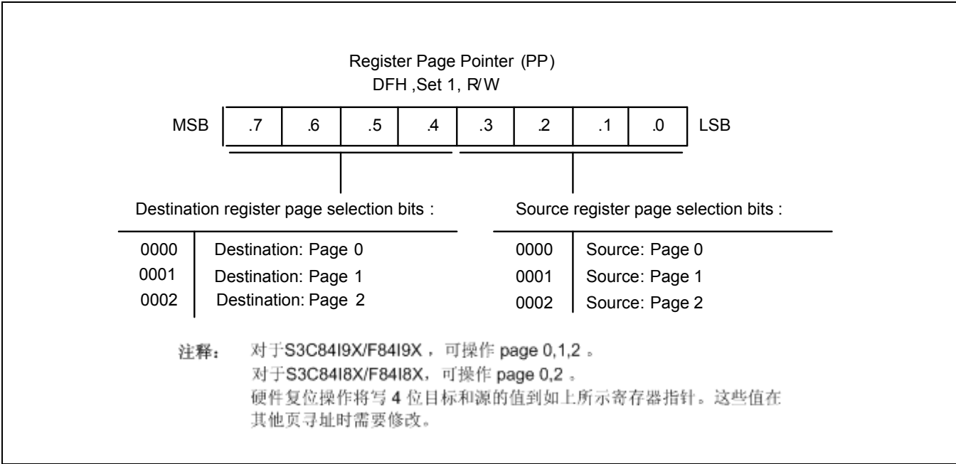
图 2-5 寄存器页面指针 (PP)
