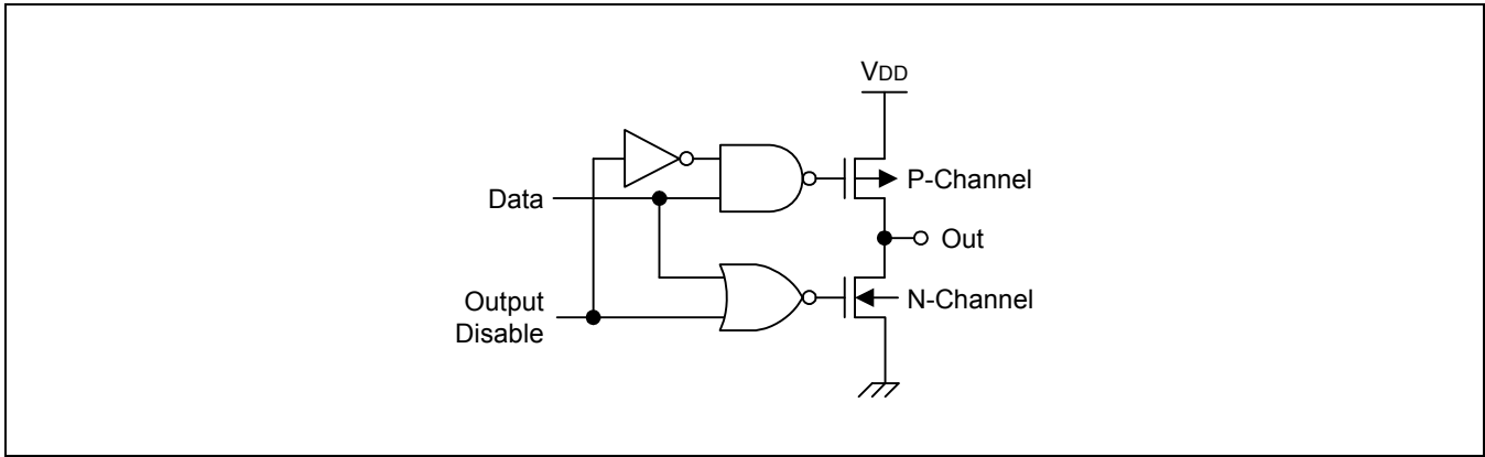
图 1-5 管脚电路类型C
