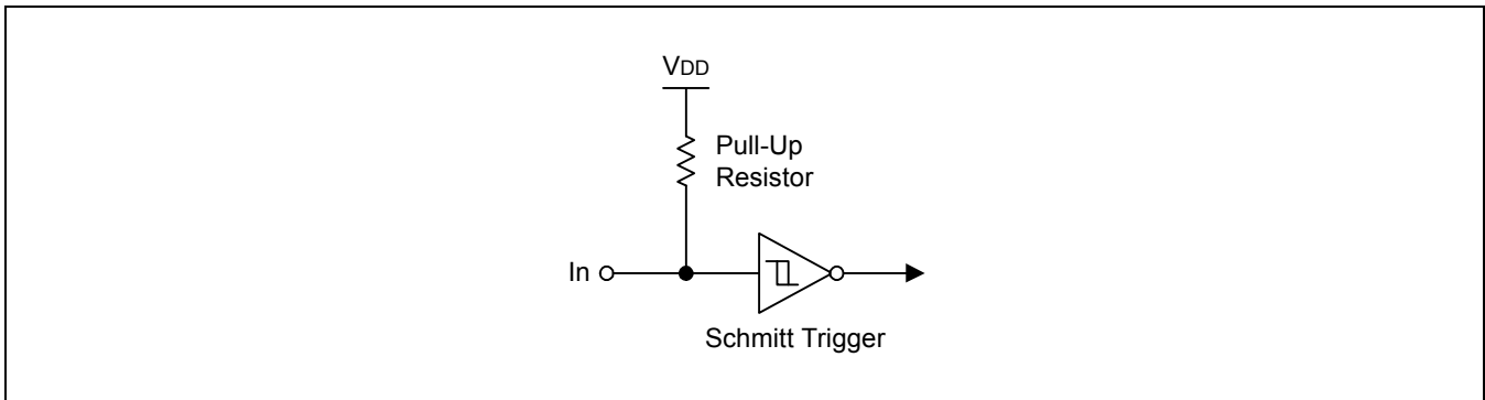
图 1-4 管脚电路类型B (nRESET)
