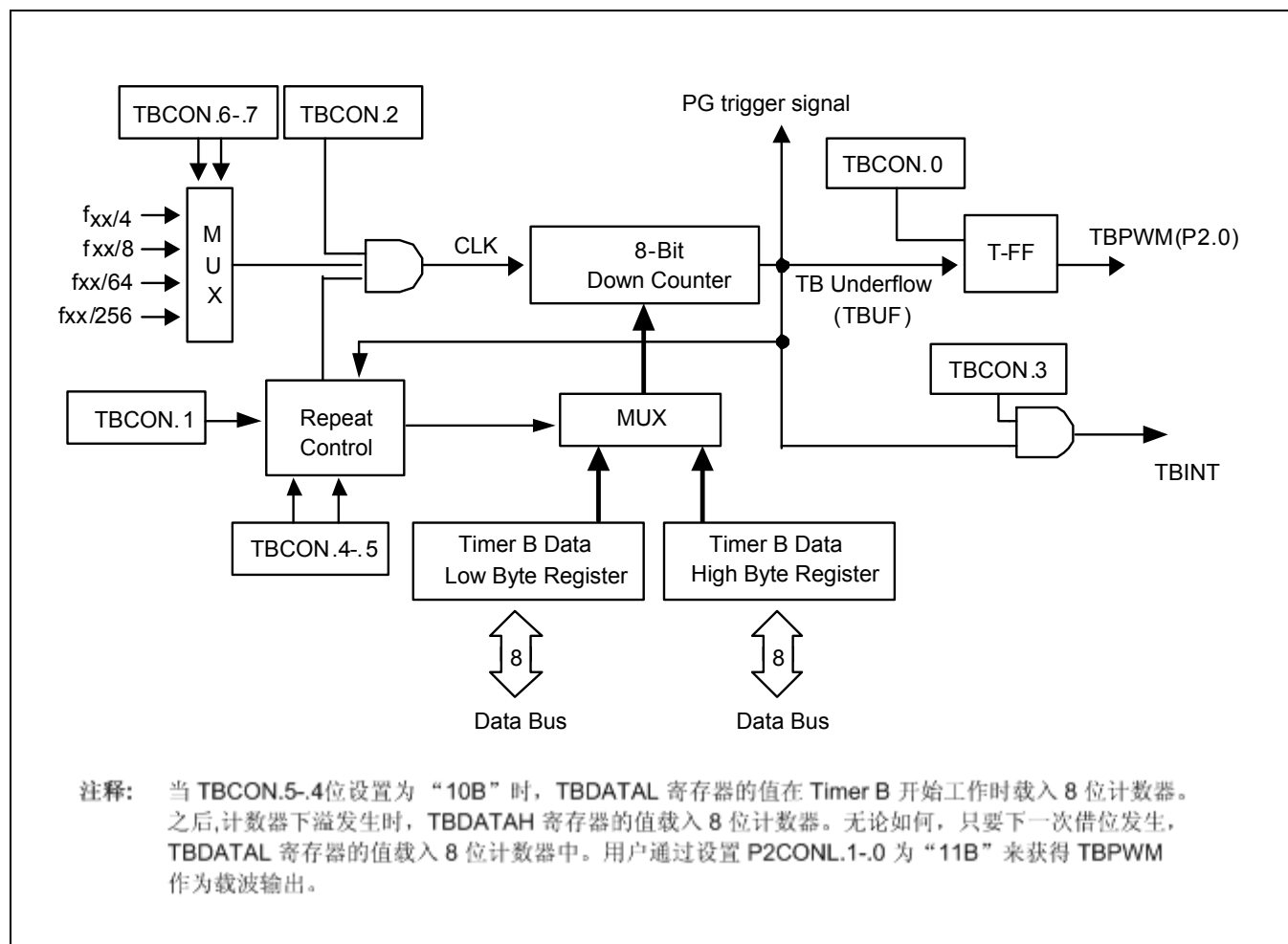
图 11-3 Timer B 功能模块框图
