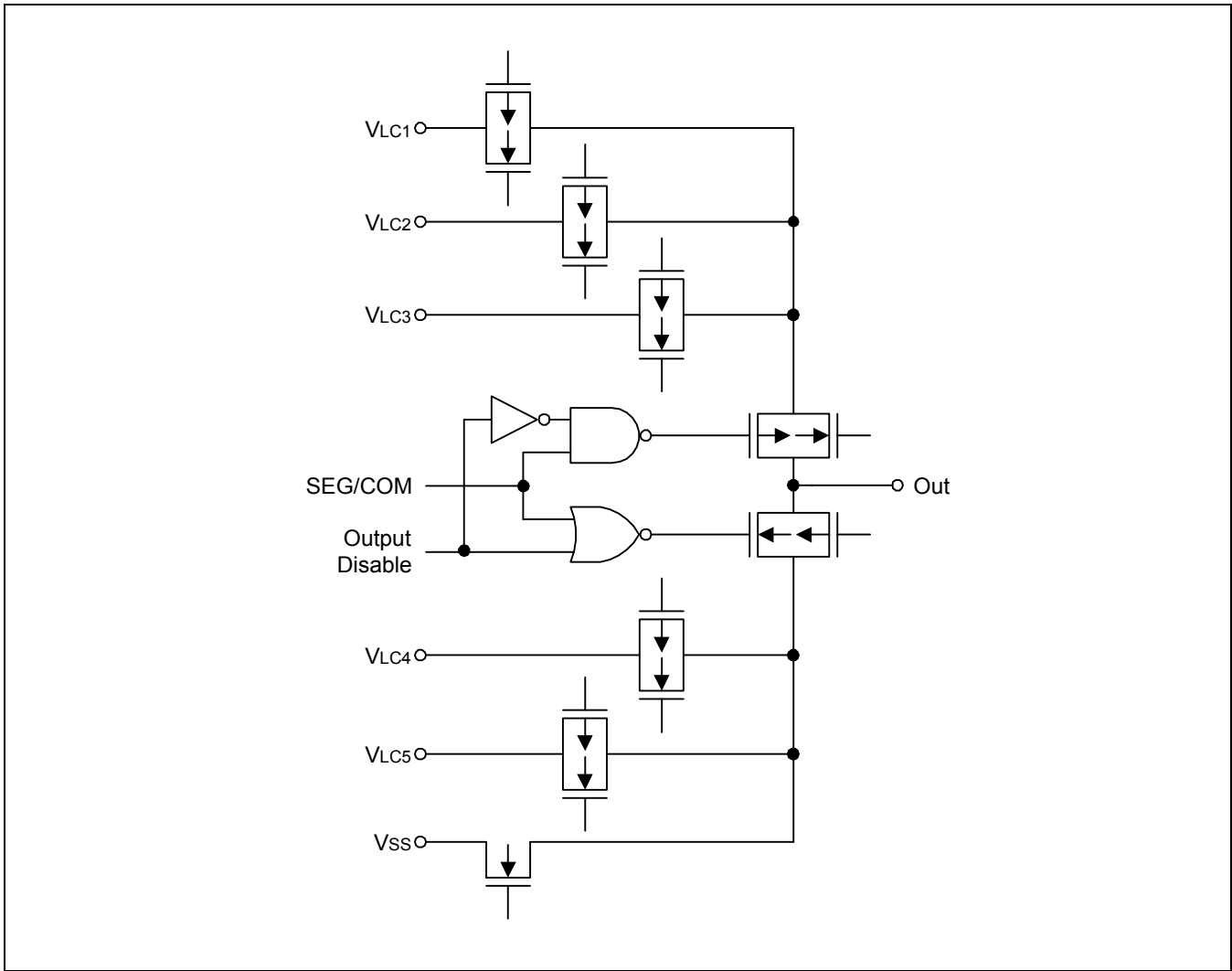
图 1-9 管脚电路类型 H-4
