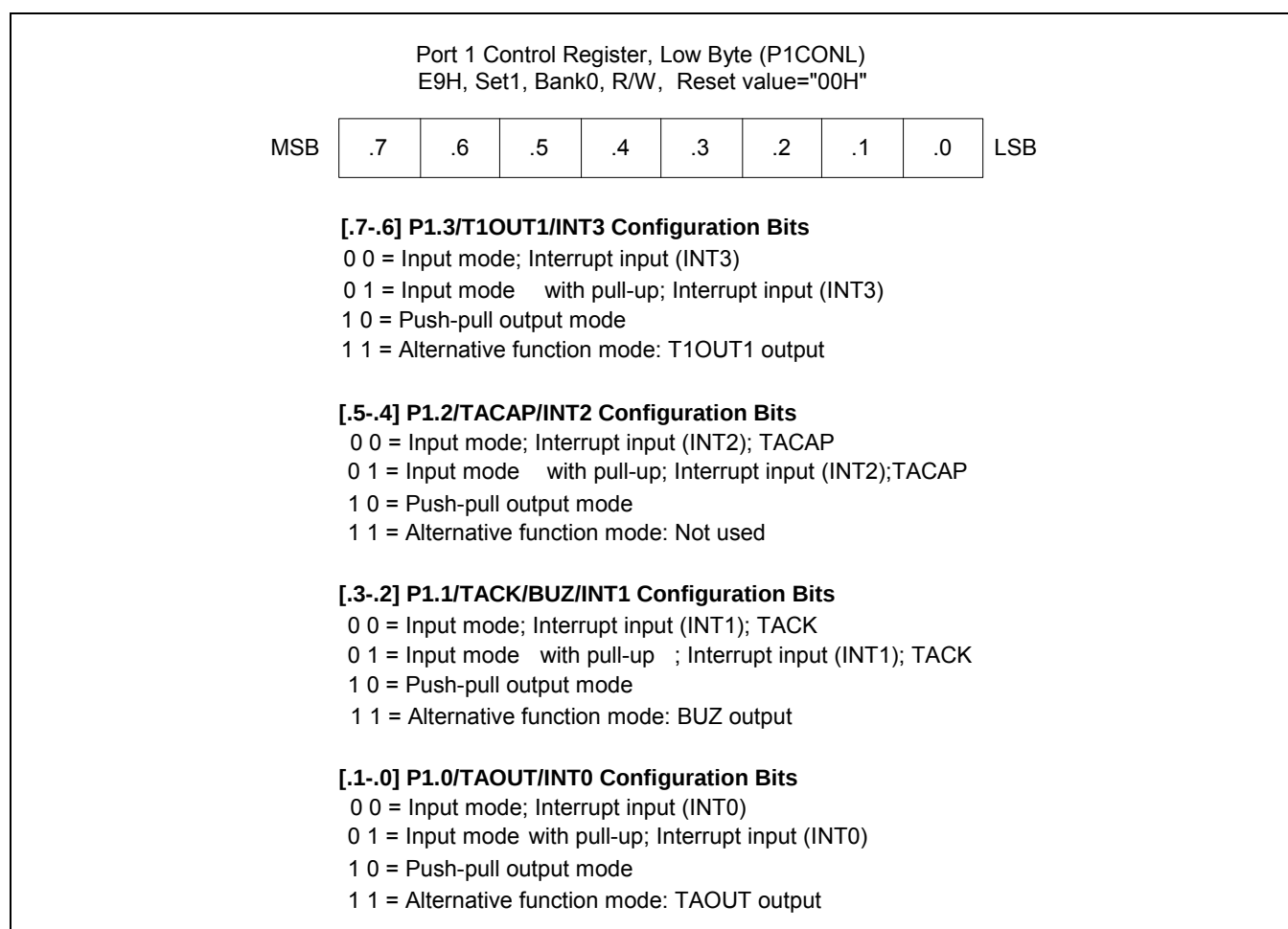
图 9-3 P1 口低字节控制寄存器 (P1CONL)
