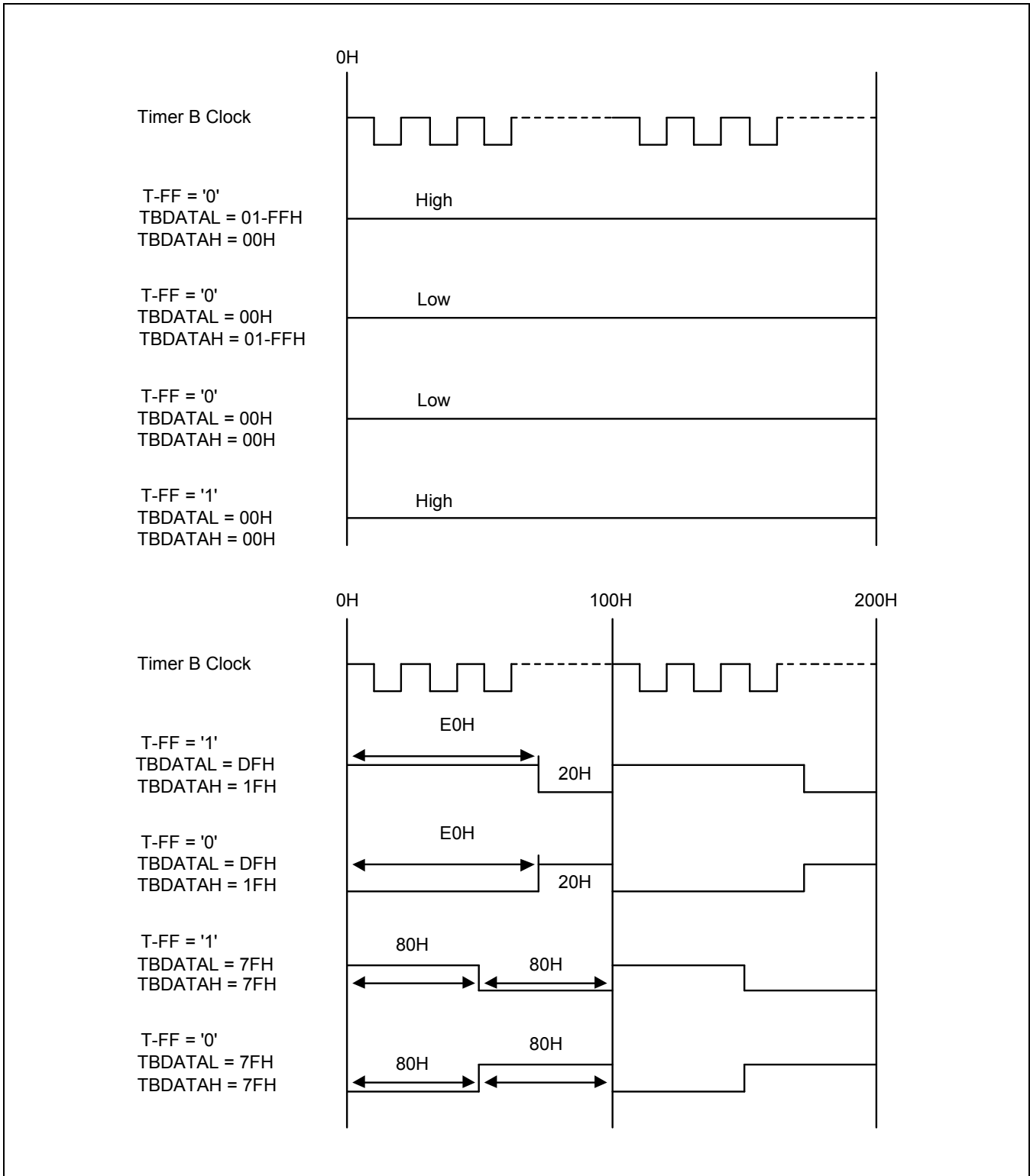
图 11-6 Timer B 在重复模式下输出触发器波形
