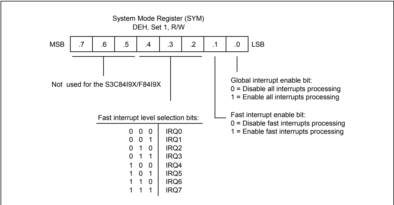
图 5-5 系统模式控制寄存器 (SYM)
