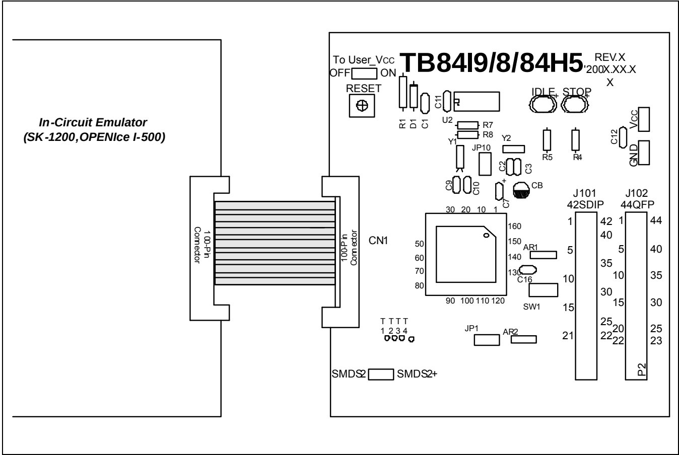
图 23-2 S3F84I9X/ S3F84I8X 目标板配置
