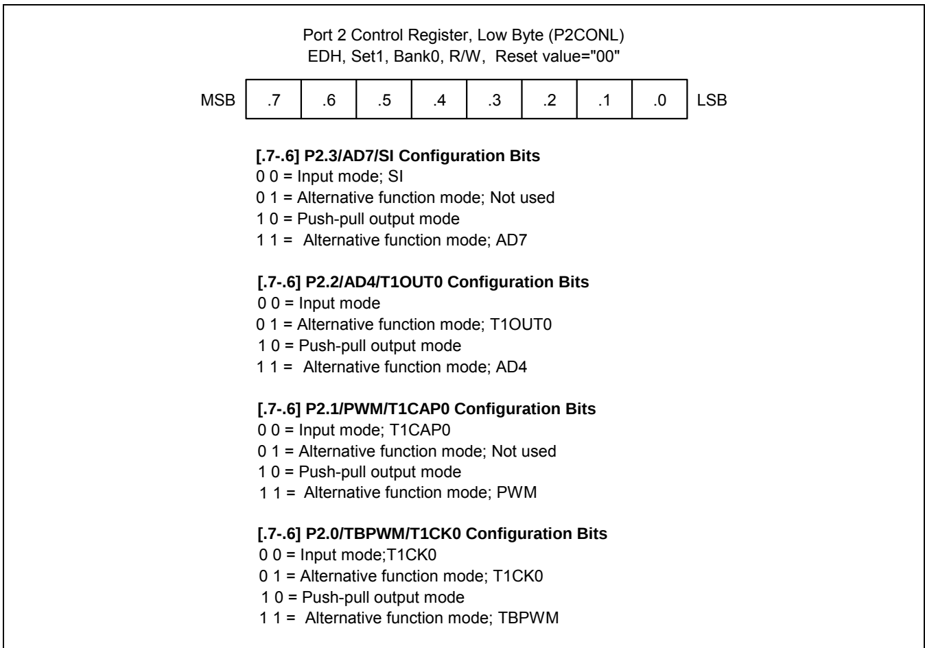
图 9-7 P2 口低字节控制寄存器 (P2CONL)
