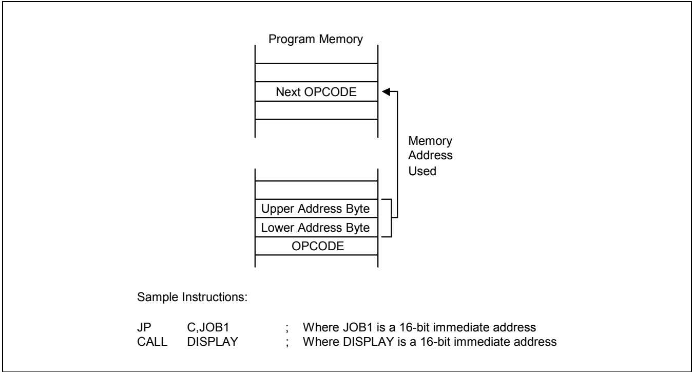
图 3-11 Call, Jump 的直接寻址
