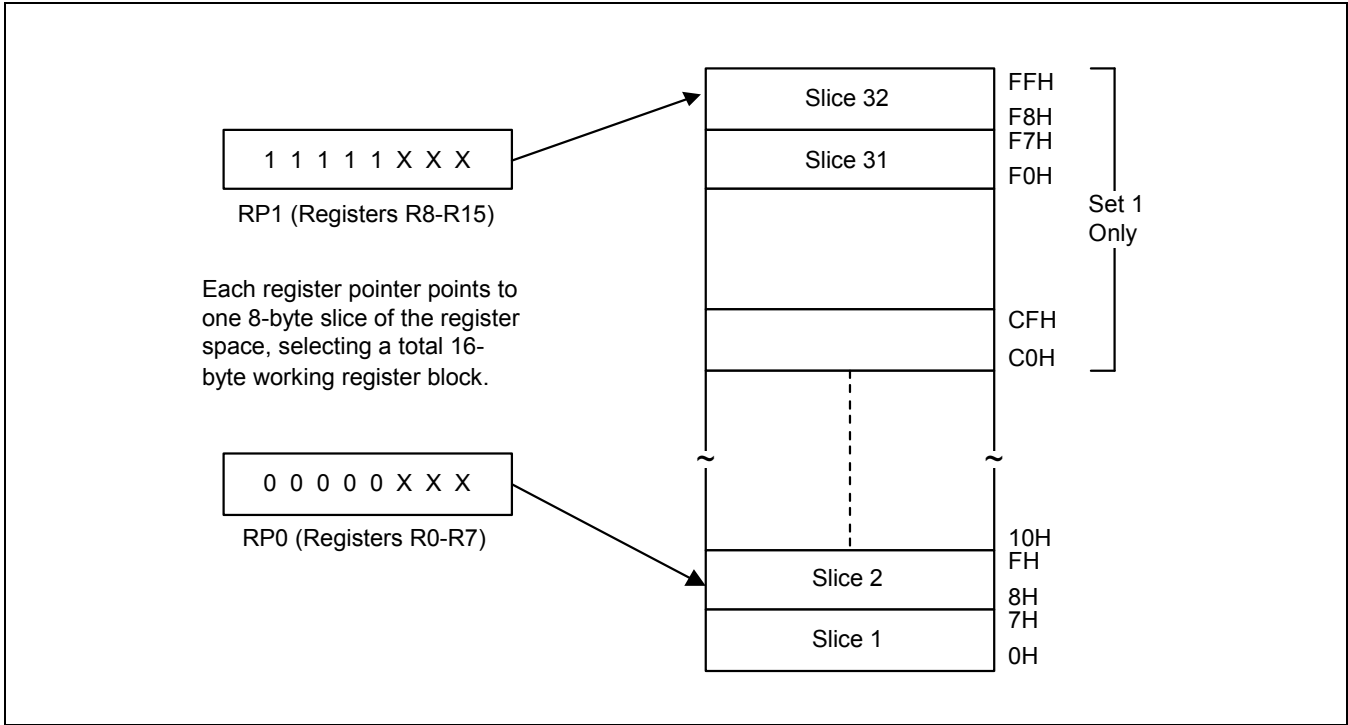
图 2-8 8 字节工作寄存器区 (Slices)
