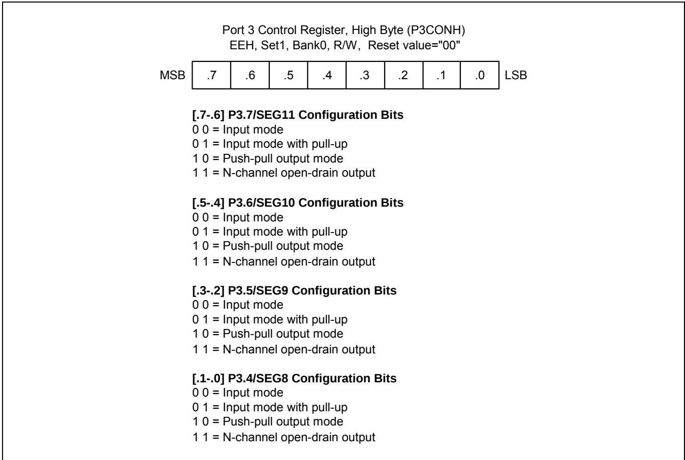
图 9-9 P3 口高字节控制寄存器 (P3CONH)
