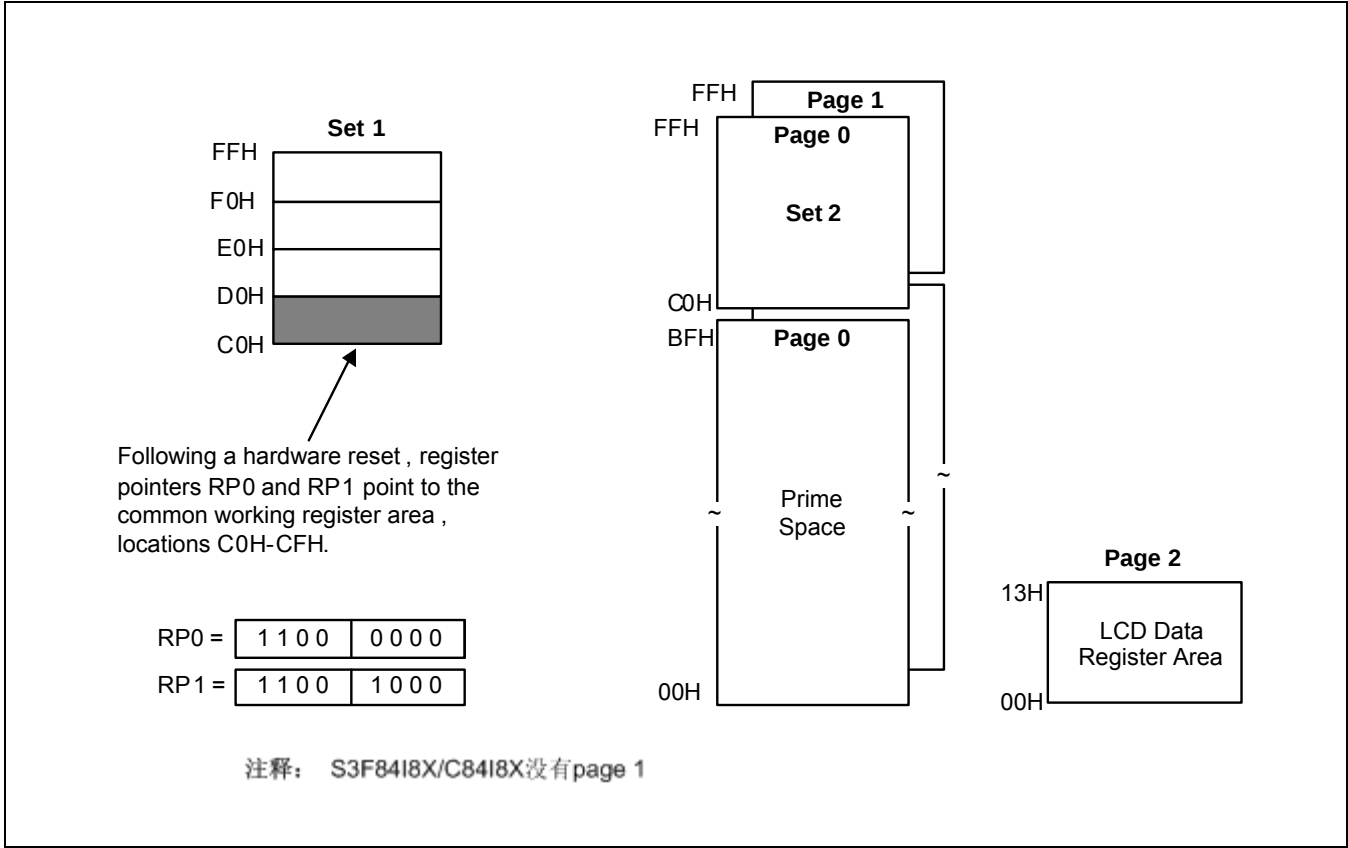
图 2-13 通用工作寄存器区
