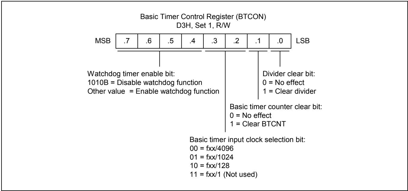
图 10-1 Basic Timer 控制寄存器 (BTCON)
