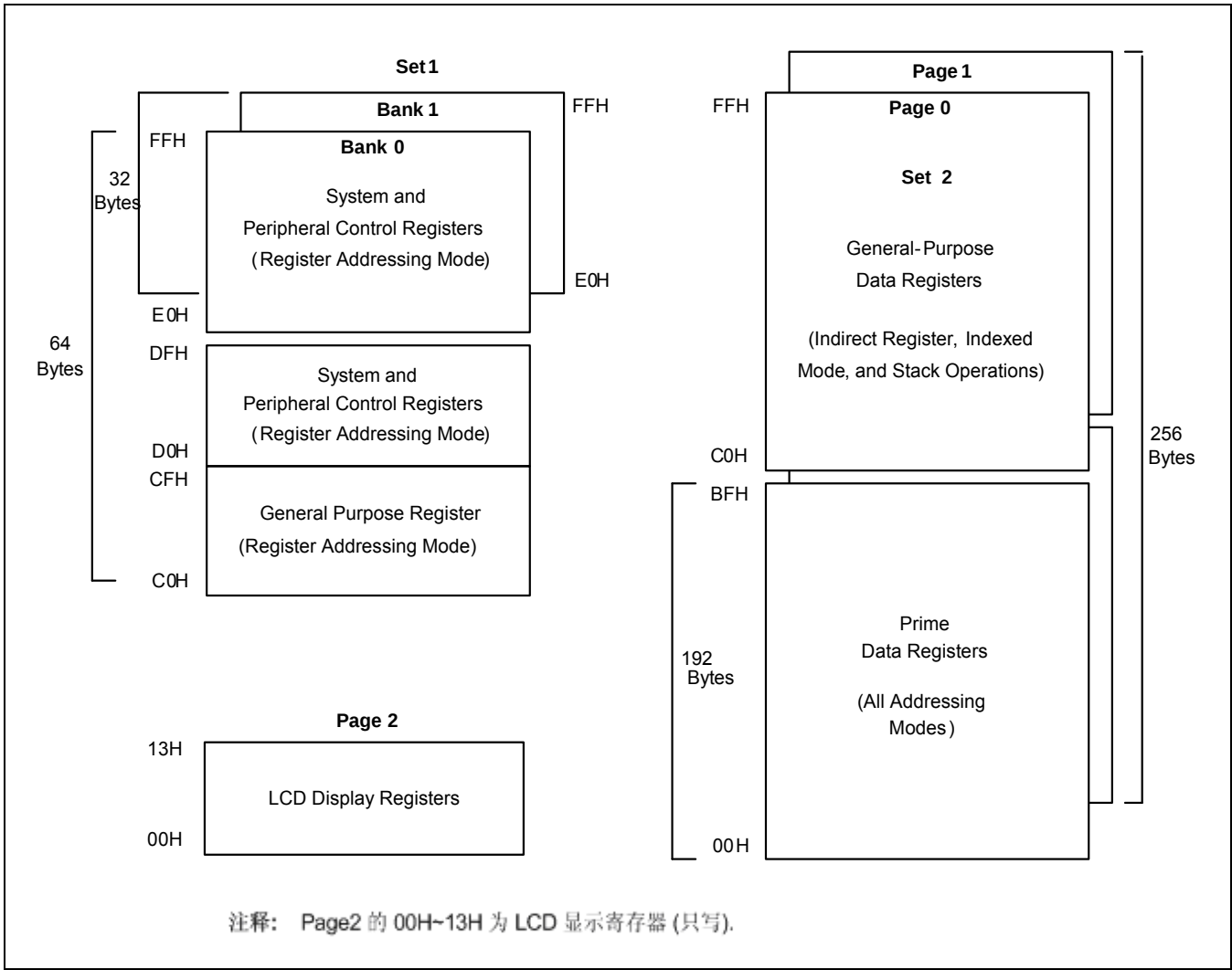
图 2-3 S3F84I9X/C84I9X 内部寄存器卷的地址空间
