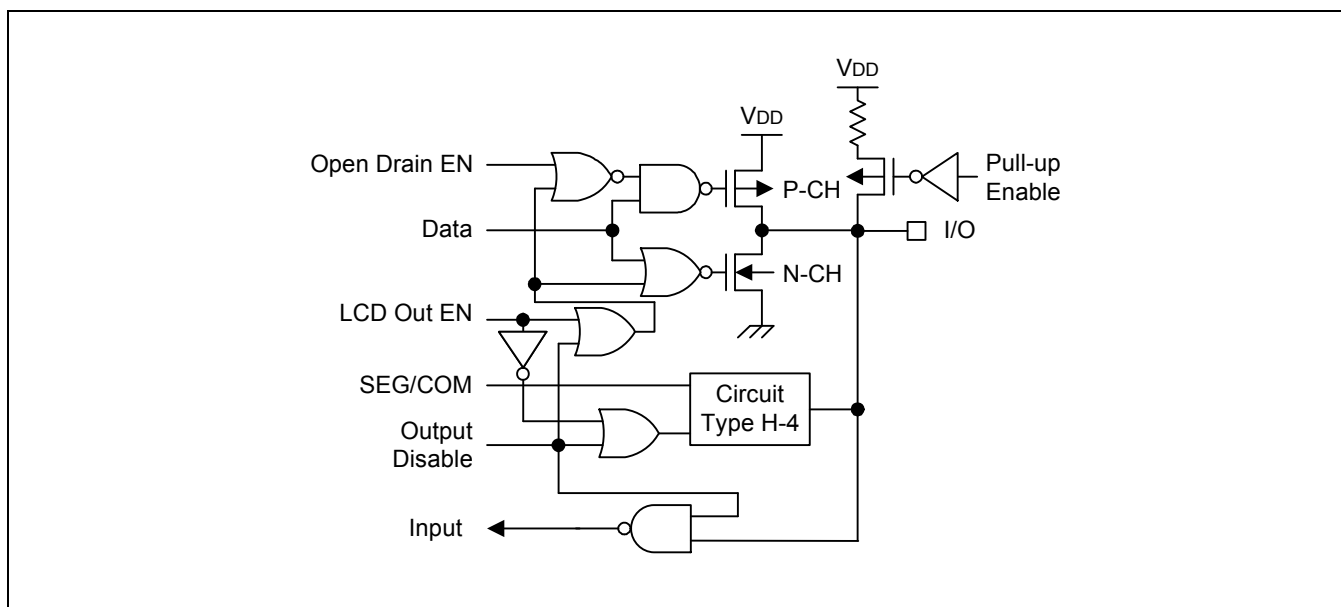
图 1-10 管脚电路类型 H-14 (P4.4-P4.7)
