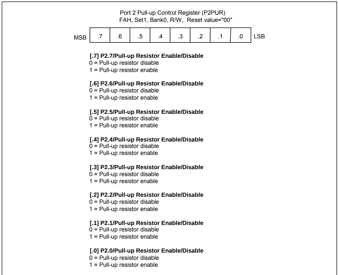
图 9-8 P2 口上拉电阻控制寄存器 (P2PUR)
