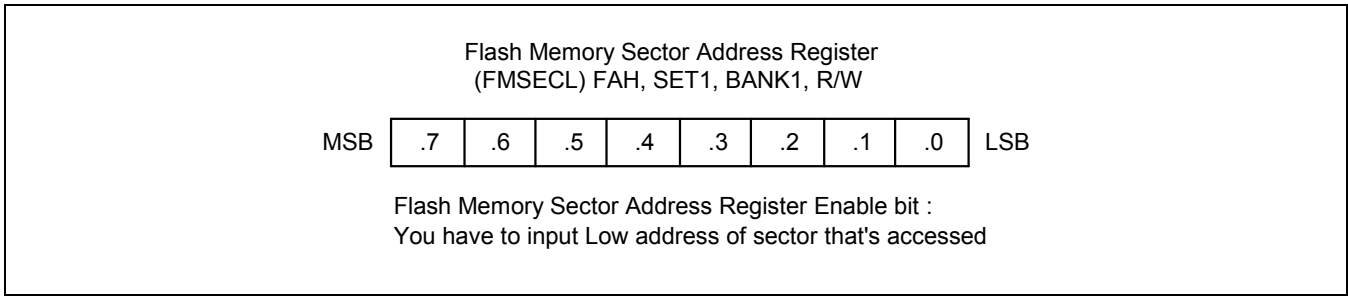
图 20-5 闪存扇区地址寄存器低字节 (FMSECL)
