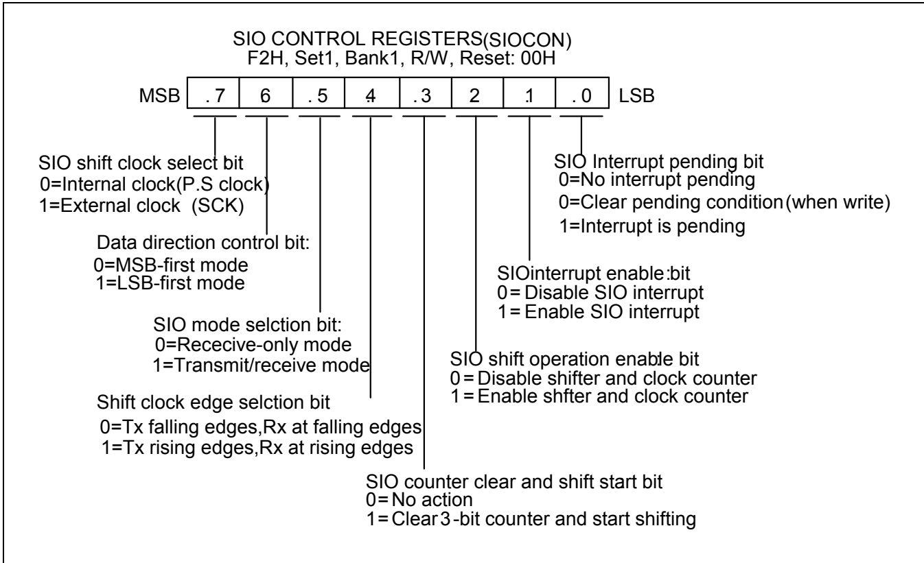
图 14-1 SIO 控制寄存器 (SIOCON)
