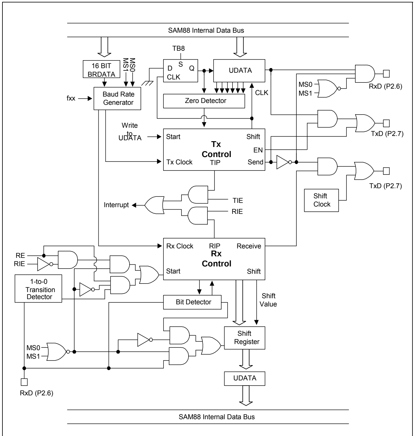
图 15-5 UART 功能模块框图
