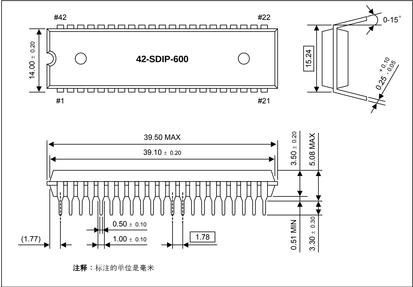
图 22-1 42-SDIP-600 封装尺寸
