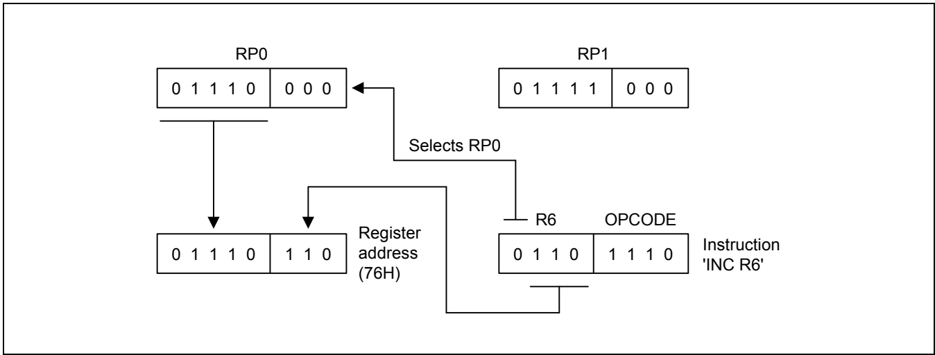
图 2-15 4 位工作寄存器寻址实例
