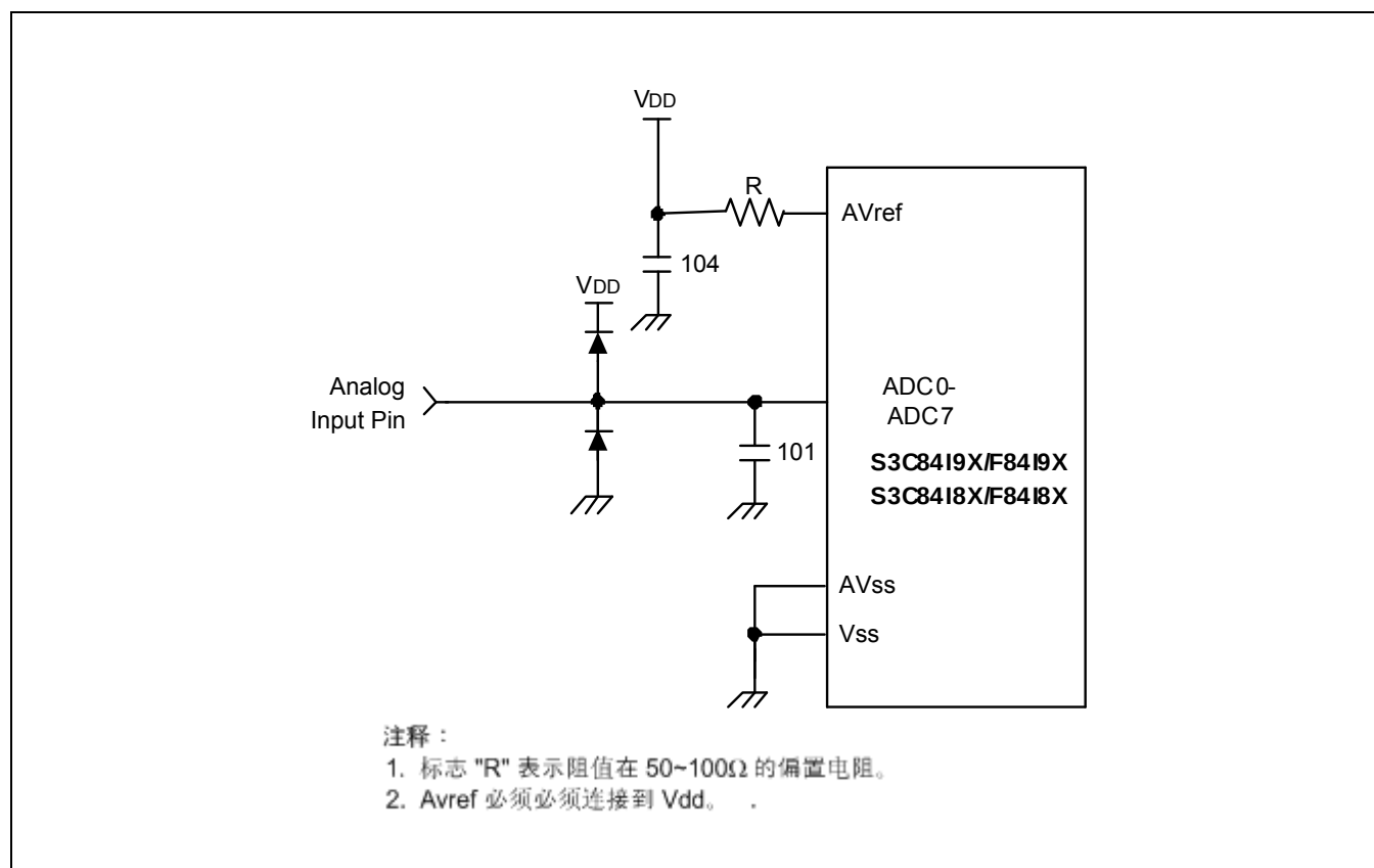
图 16-5 推荐高精度 A/D 转换电路
