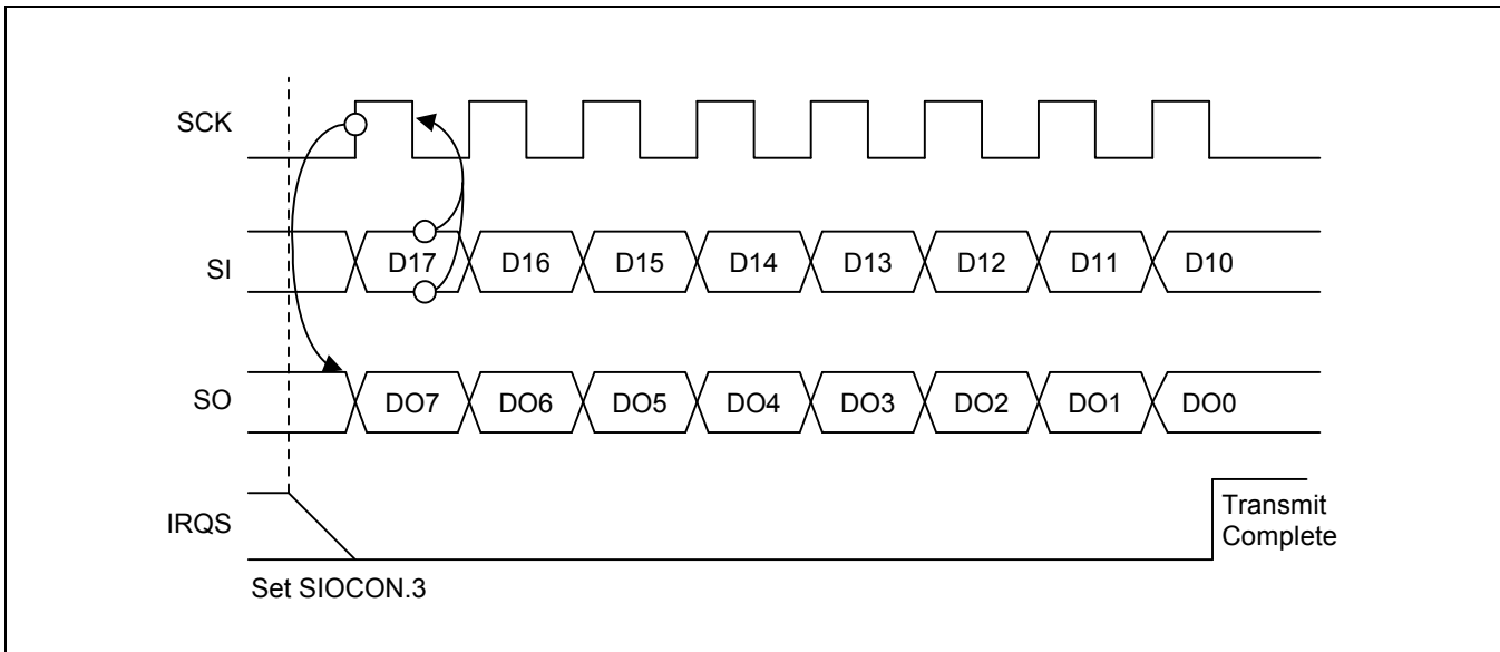
图 14-5 SIO 发送/接收模式 (上升沿发送, SIOCON.4 = 1)
