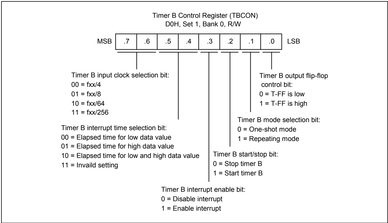
图 11-4 Timer B 控制寄存器 (TBCON)
