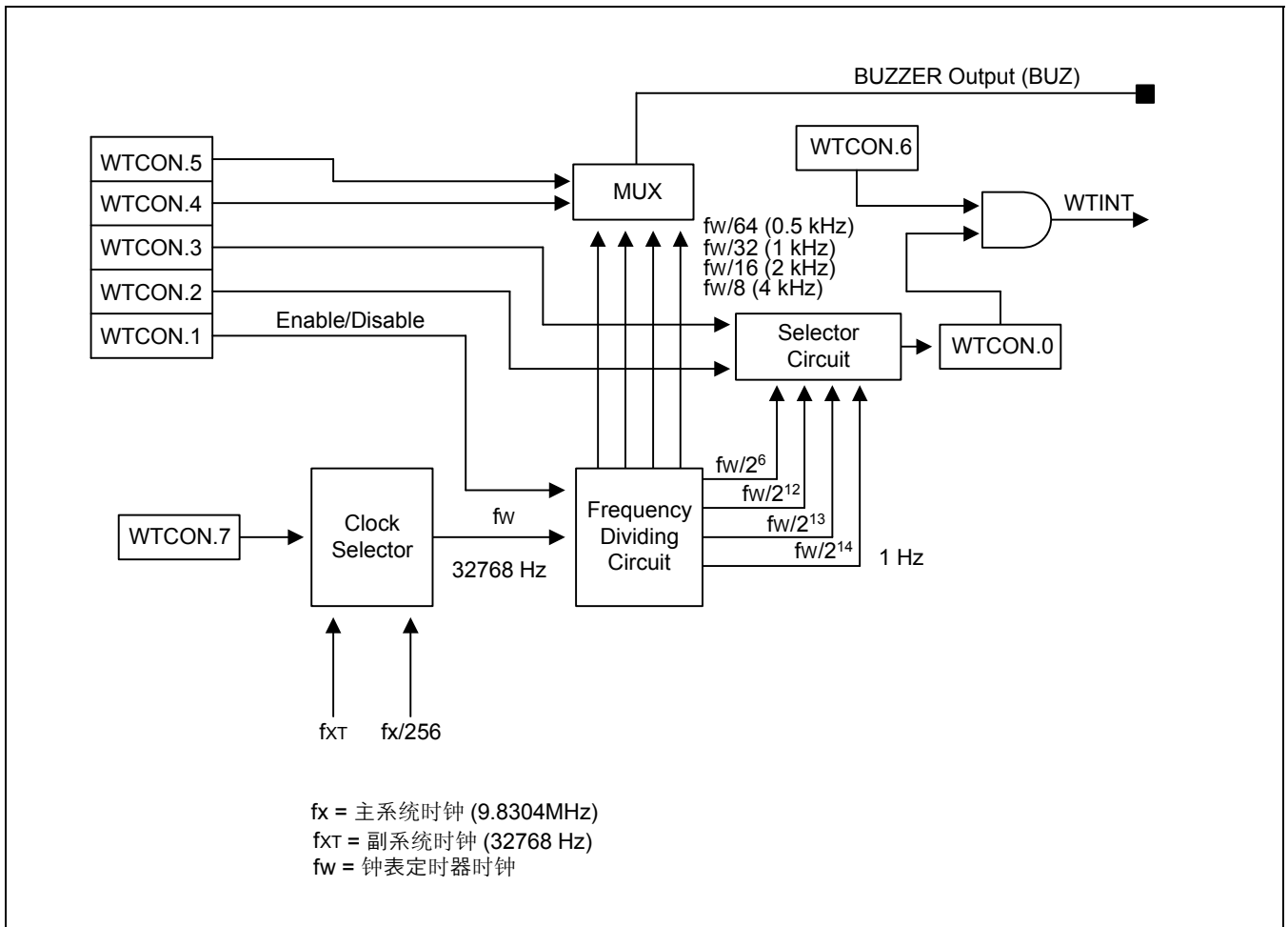
图 17-1 钟表定时器电路框图
