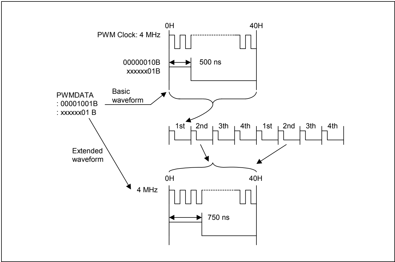
图 13-2 PWM ‘延伸’ 波形 (10位)
