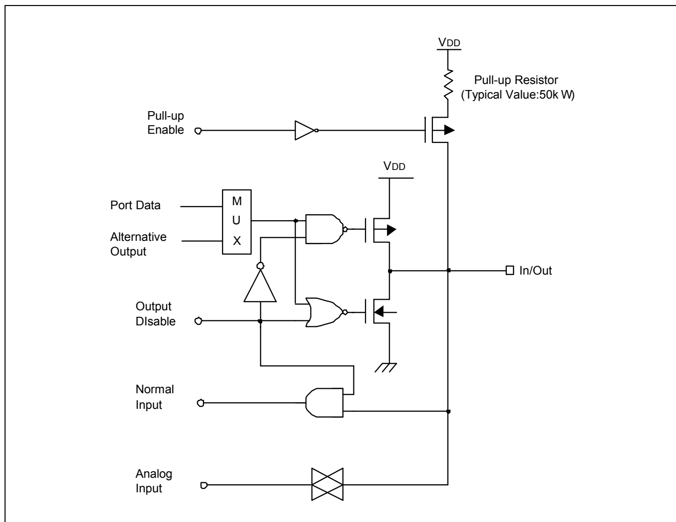
图 1-8 管脚电路类型 E (P2.2-P2.3)
