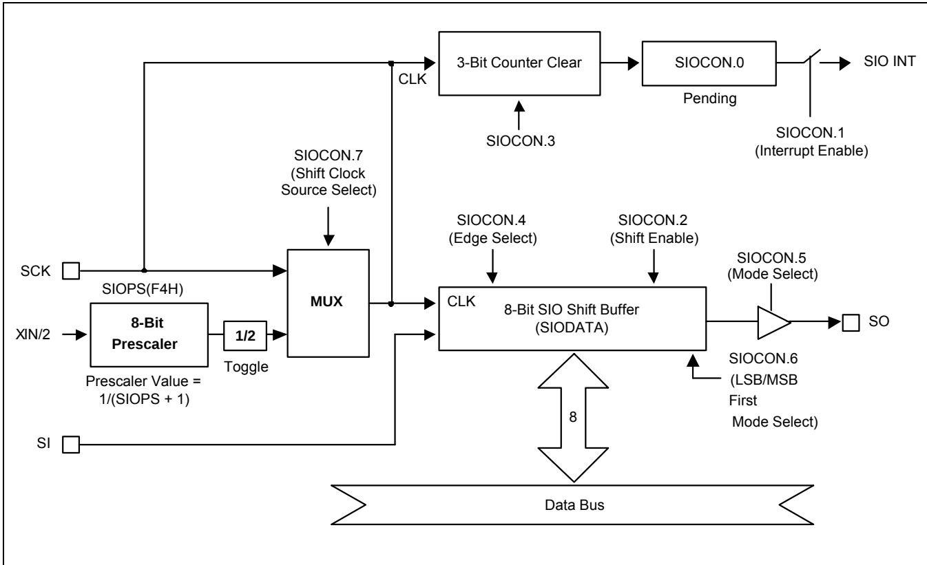
图 14-3 SIO 功能模块框图
