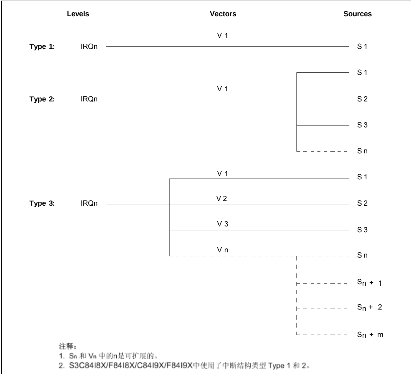
图 5-1 S3C8-系列的中断类型
