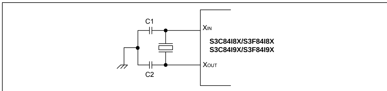
图 7-1 主振荡电路 (石英/陶瓷晶振)
