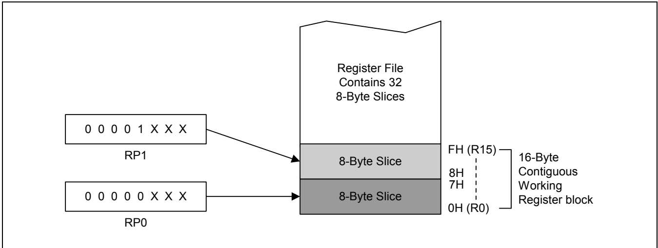
图 2-9 相邻的16 字节工作寄存器块
