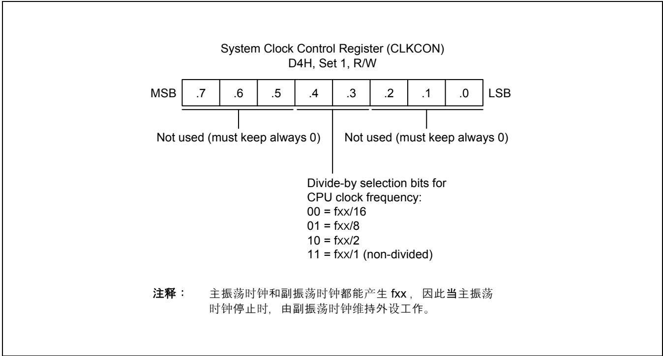
图 7-4 系统时钟控制寄存器 (CLKCON)
