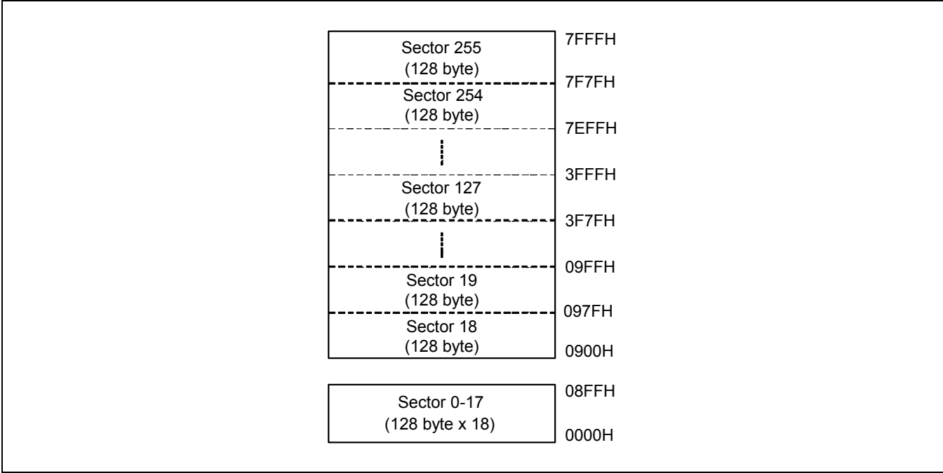
图 20-3 用户编程模式下的扇区
