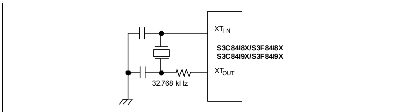
图 7-2 副振荡电路 (石英晶振)
