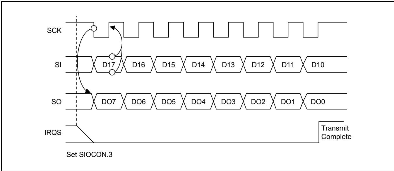
图 14-4 SIO 发送/接收模式 (下降沿发送, SIOCON.4 = 0)
