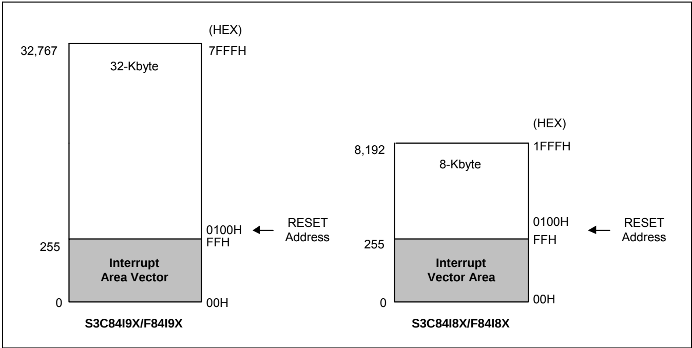
图 5-3 ROM中断向量地址区
