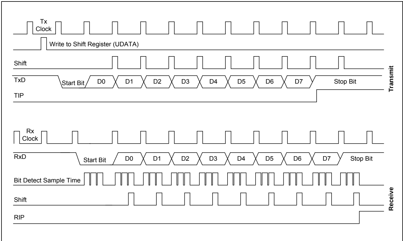
图 15-7 UART Mode 1 模式运行时序图
