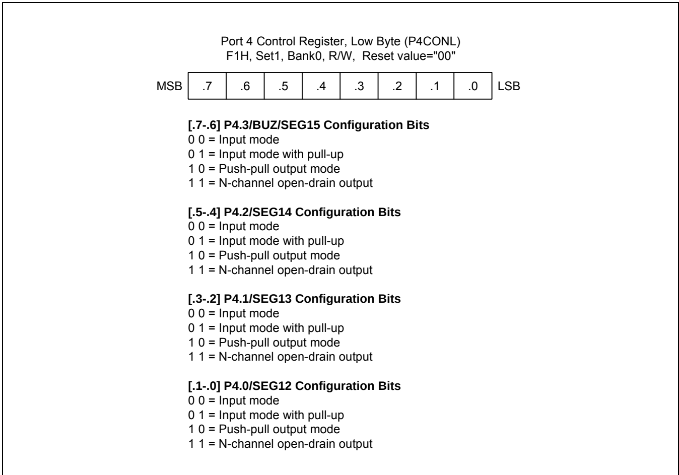
图 9-12 P4 口低字节控制寄存器 (P4CONL)
