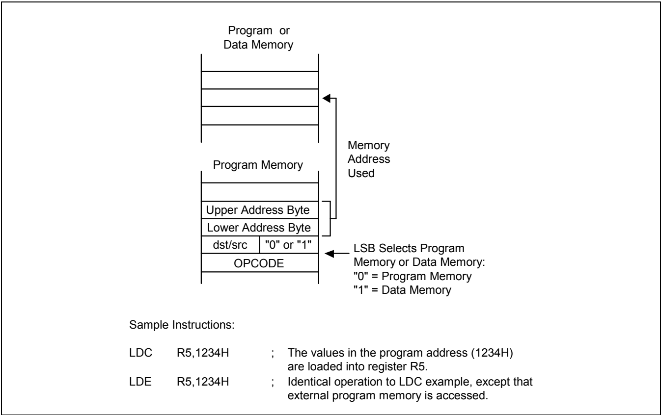
图 3-10 Load 指令的直接寻址
