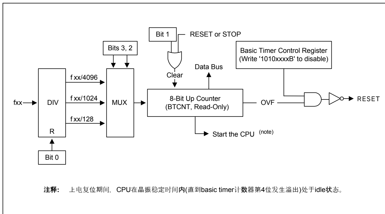
图 10-2 Basic Timer 方框图
