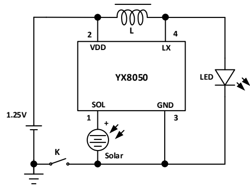
图 6. 推荐接法 2
