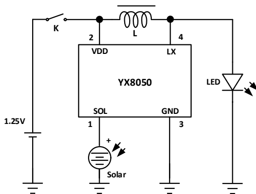
图 5. 推荐接法 1
