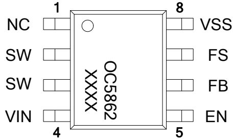
ESOP8
