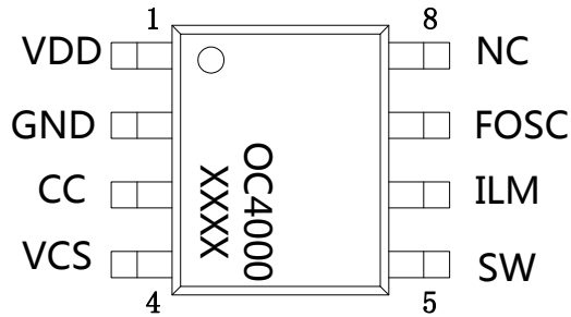
ESOP8
